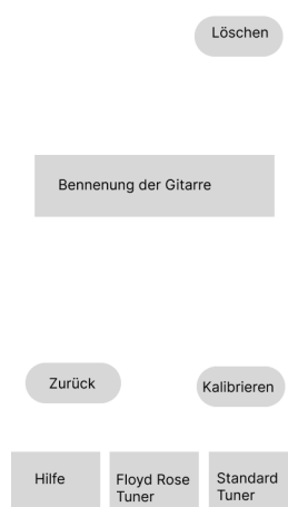
Abbildung 26: Wireframe: Gitarre bearbeiten
