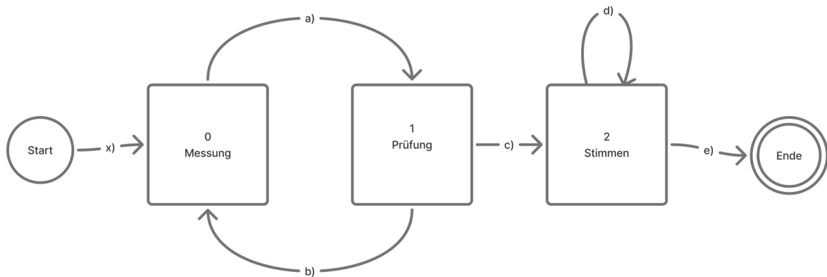
Abbildung 47: Zustandsdiagramm: Stimmlogik
