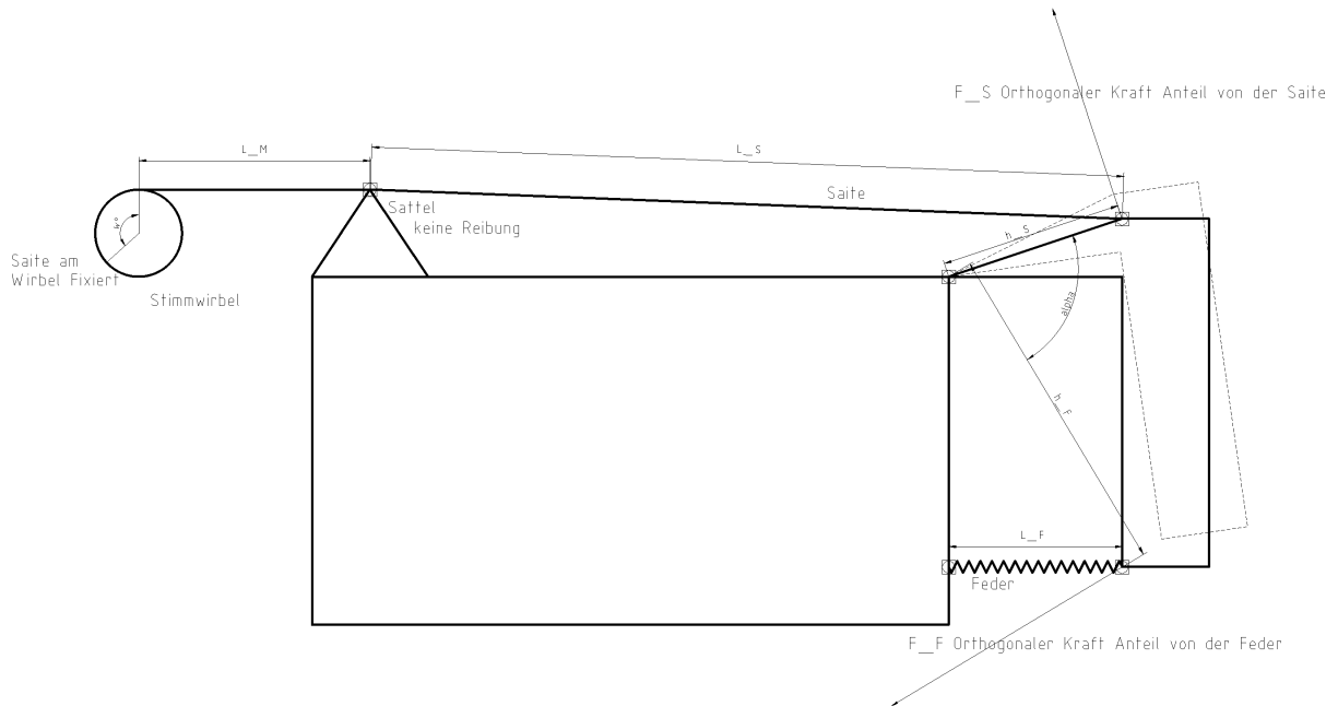
Abbildung 19: Querschnittsmodell des physikalischen Modells der Floyd-Rose-Brücke
