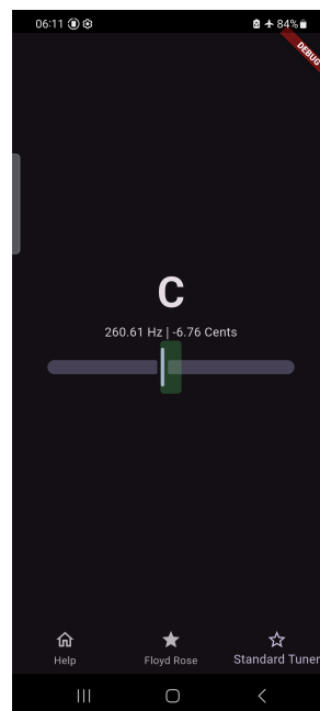
Abbildung 44: Design: Standard-Stimmgerät
