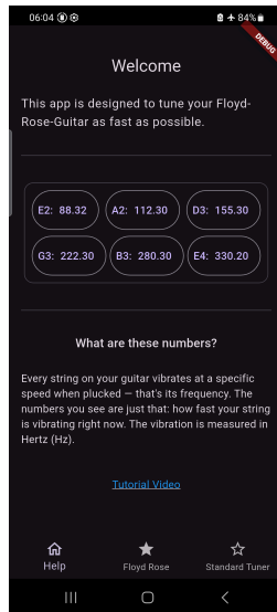
Abbildung 33: Design: Hilfsseite
