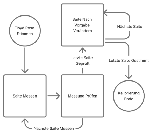
Abbildung 22: Interaktionsdesign – Stimmprozess
