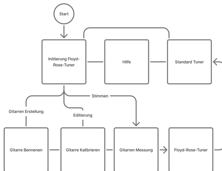
Abbildung 20: Interaktionsdesign – Navigation
