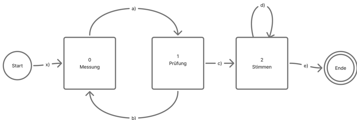
Abbildung 46: Zustandsdiagramm: Stimmlogik
