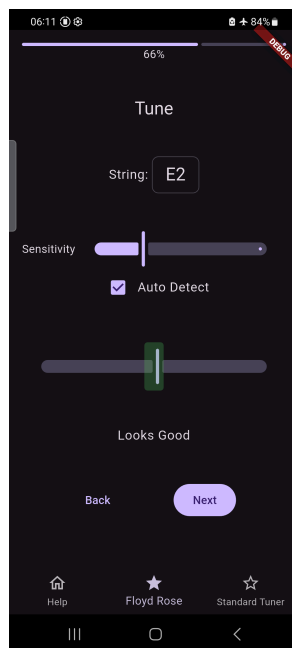
Abbildung 43: Design: Floyd-Rose-Tuner
