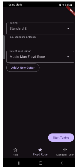
Abbildung 34: Design: Startseite
