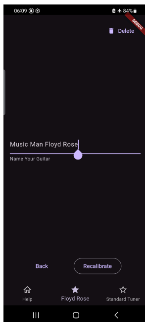
Abbildung 42: Design: Rekalibrieren
