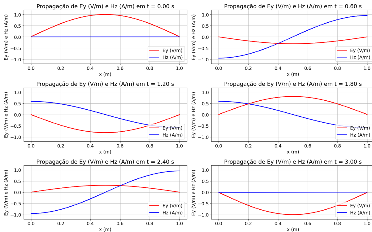
Figura 13 – Propagação de E_y e H_z ao longo do tempo - fluxo upwind.
