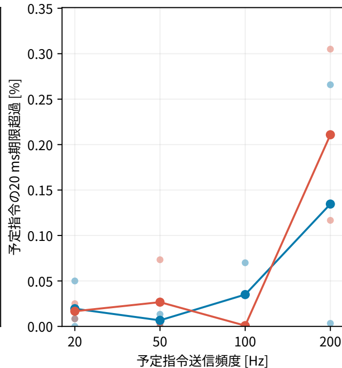
ESP-NOW連続指令：未送信・欠落も期限超過へ含める / 19試行・条件ごと2〜3反復 大きい点は統合p99／期限超過・最大途絶・平均実受信、小さい点は各反復
