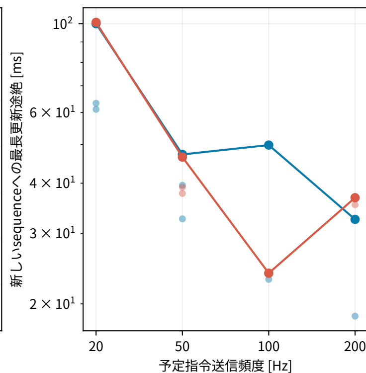
ESP-NOW連続指令：未送信・欠落も期限超過へ含める / 19試行・条件ごと2〜3反復 大きい点は統合p99／期限超過・最大途絶・平均実受信、小さい点は各反復
