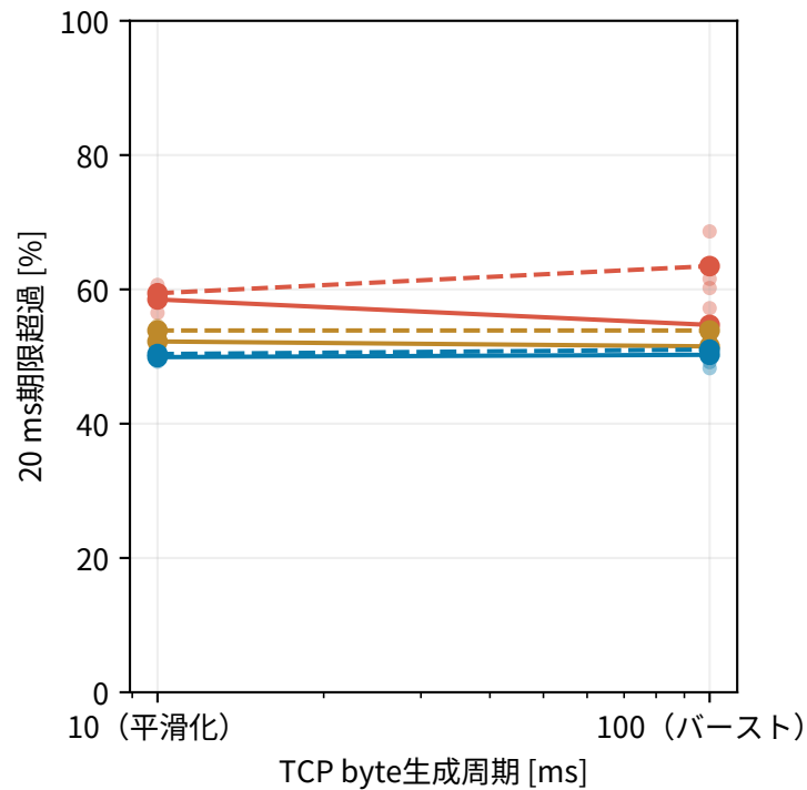
同じ平均要求量で生成周期を変更：実受信量と指令品質を同時に評価
