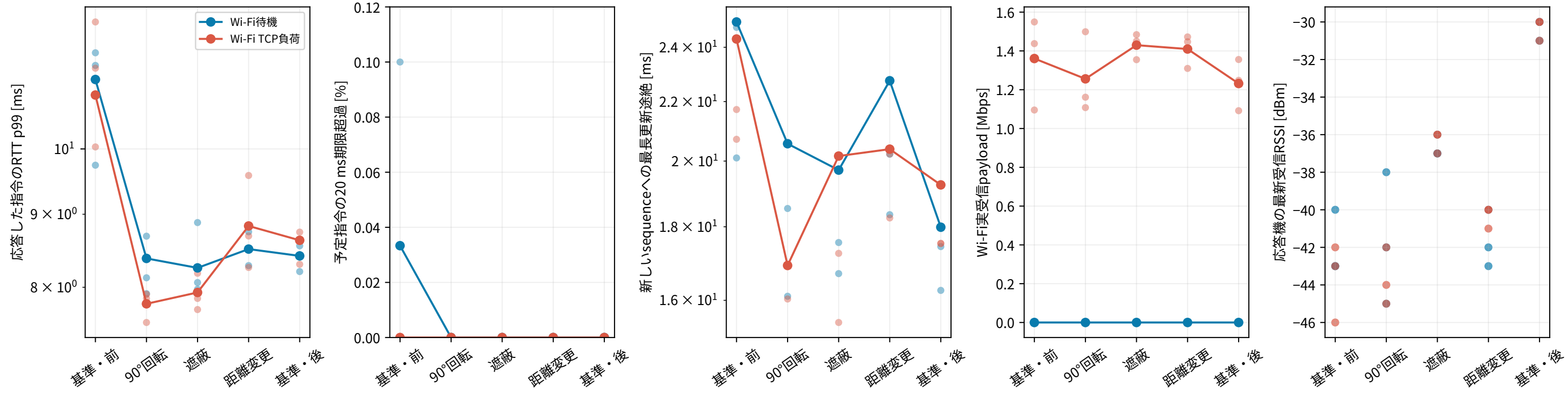
手動配置比較：ESP-NOW Ch6・100 Hz・各10秒、別系統Wi-Fi Ch6 大きい点は統合p99／期限超過・最大途絶・平均実受信、RSSIは各反復の終了読み出し
