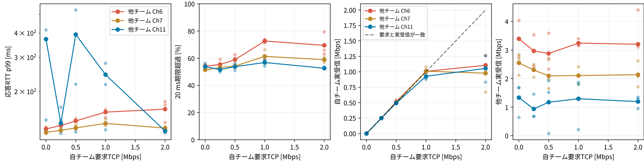
TCP流量制限：他チームに飽和TCPを要求（実受信0は0試行） | 大きい点は統合値、小さい点は各反復
