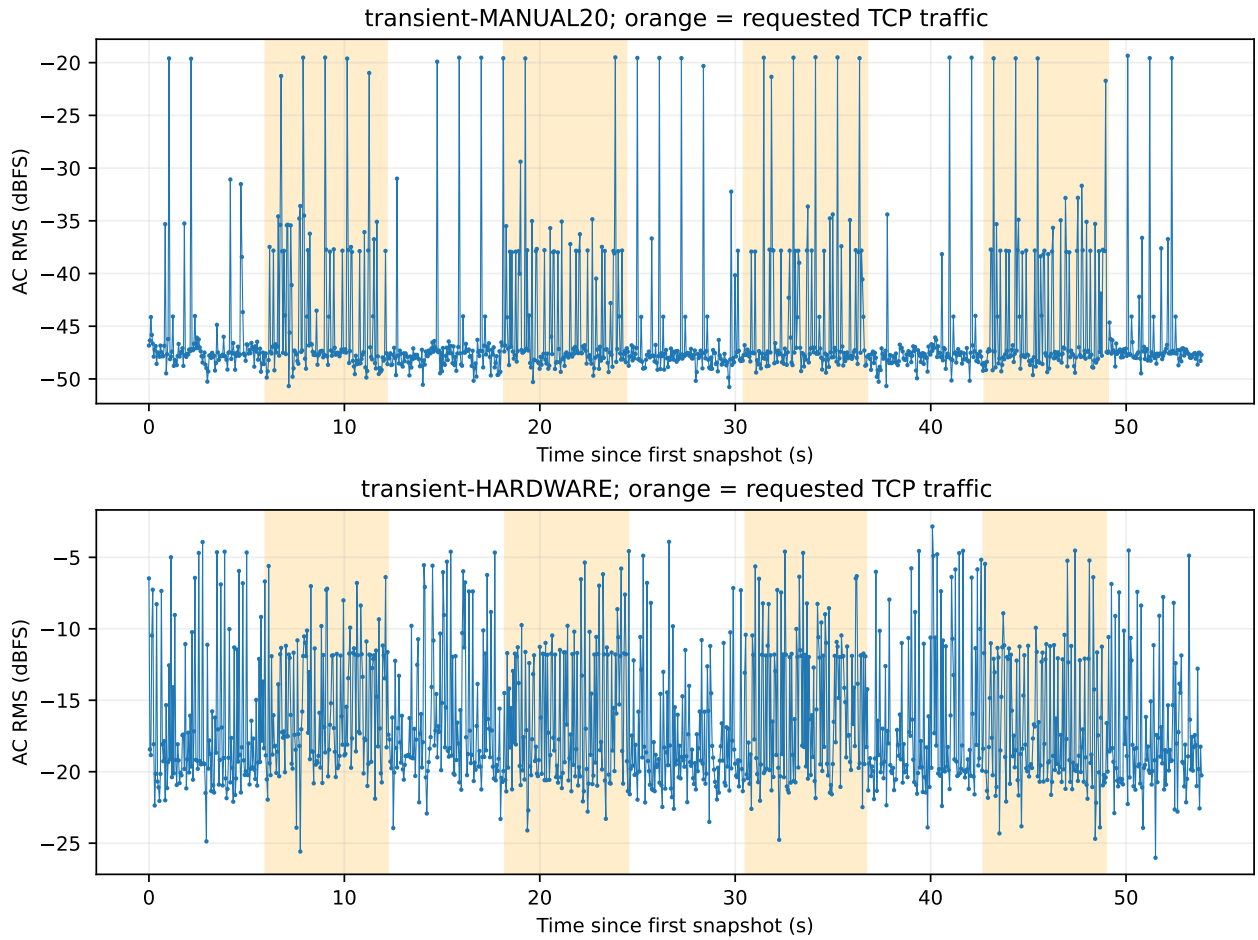
図 28 全帯域 RMS の負荷過渡。橙色は TCP を要求した時間で、各パケットの実際の送信時刻ではない。
