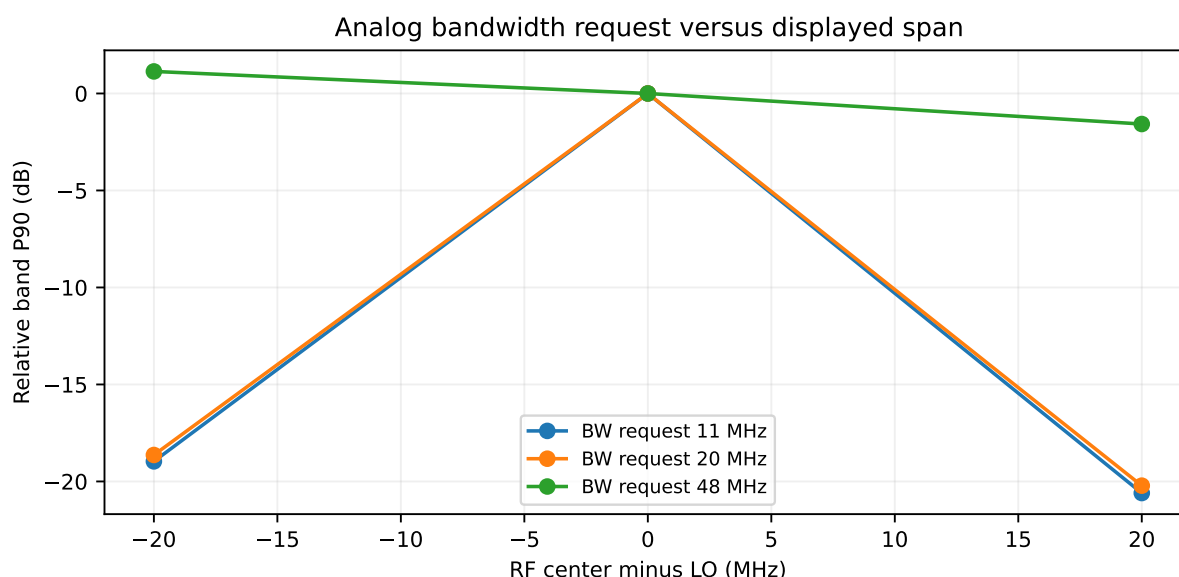
図 26 11・20・48 MHz 帯域要求での固定 RF 帯域応答。48 MHz のみ 2 反復で、反復 1 を表示。各帯域の中央 LO 条件で規格化した。
