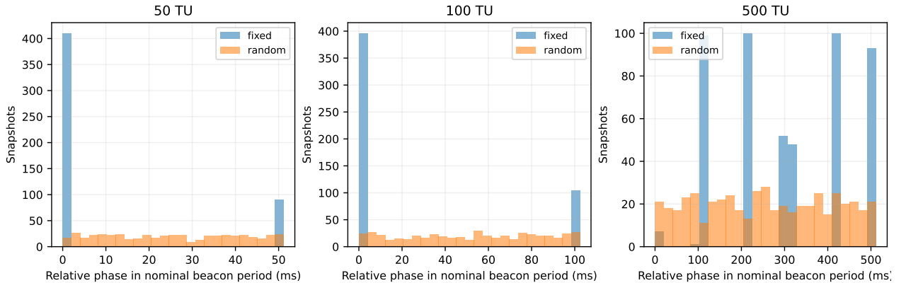
図 23 名目ビーコン周期に対する取得位相。原点は各条件の最初の取得。絶対的なビーコン到着位相やパケット捕捉率の図ではない。
