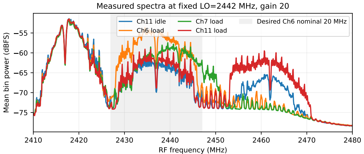
図3 独立 AP 比較の実測平均スペクトル。主 AP は Ch6 で固定。灰色は主 AP の名目 20 MHz 範囲。外来信号と受信機の周波数応答も含む。
