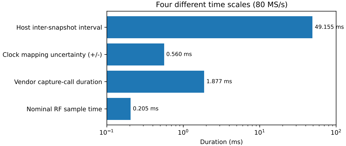
図 20 別々の意味を持つ 4 種類の時間。対数軸。処理区間と名目 RF 時間を同一視しない。
