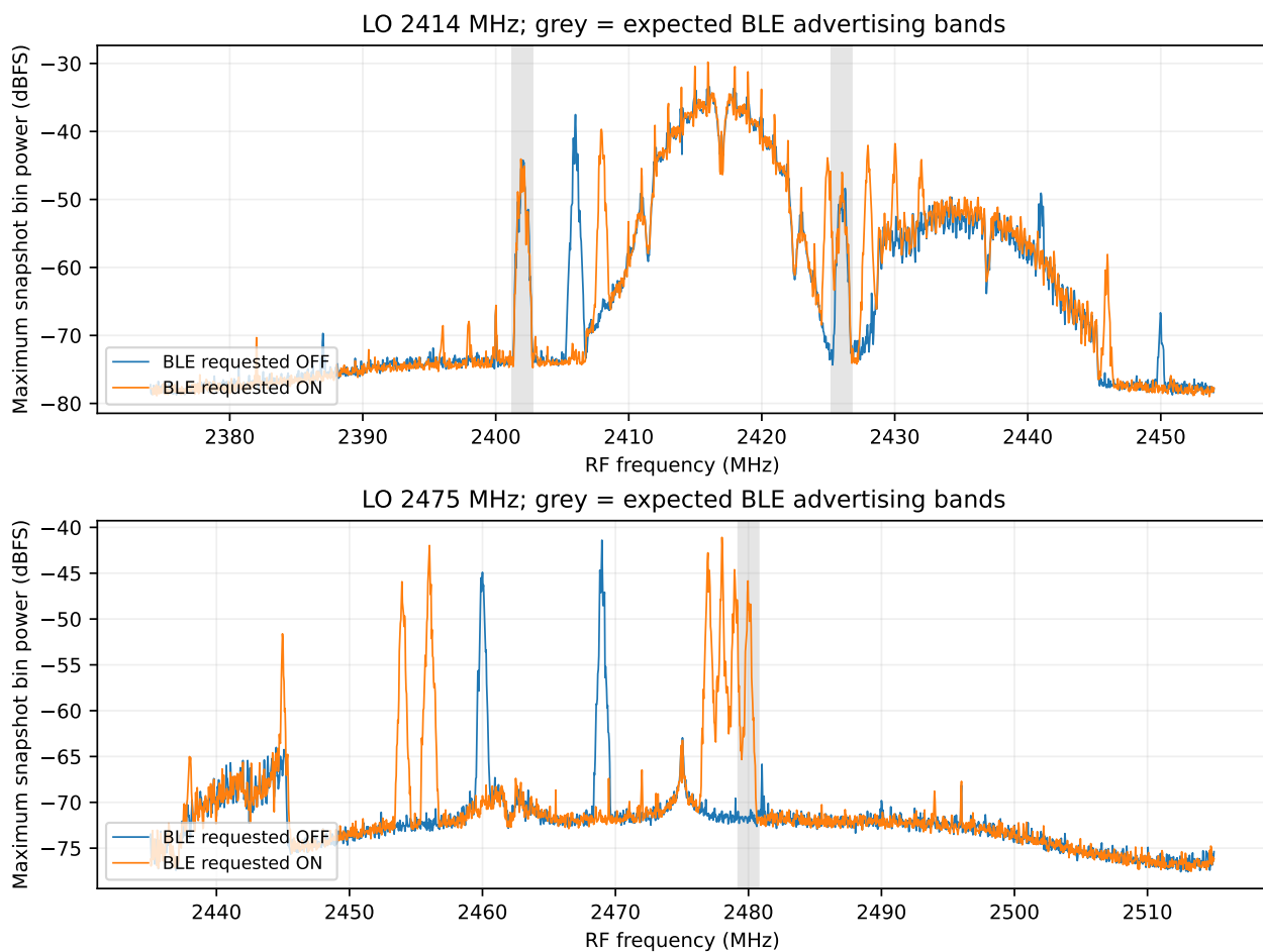
図 31 BLE ON/OFF の最大スナップショット電力。灰色は legacy 広告周波数付近。Wi-Fi 管理通信や他の Bluetooth 送信機も存在する。
