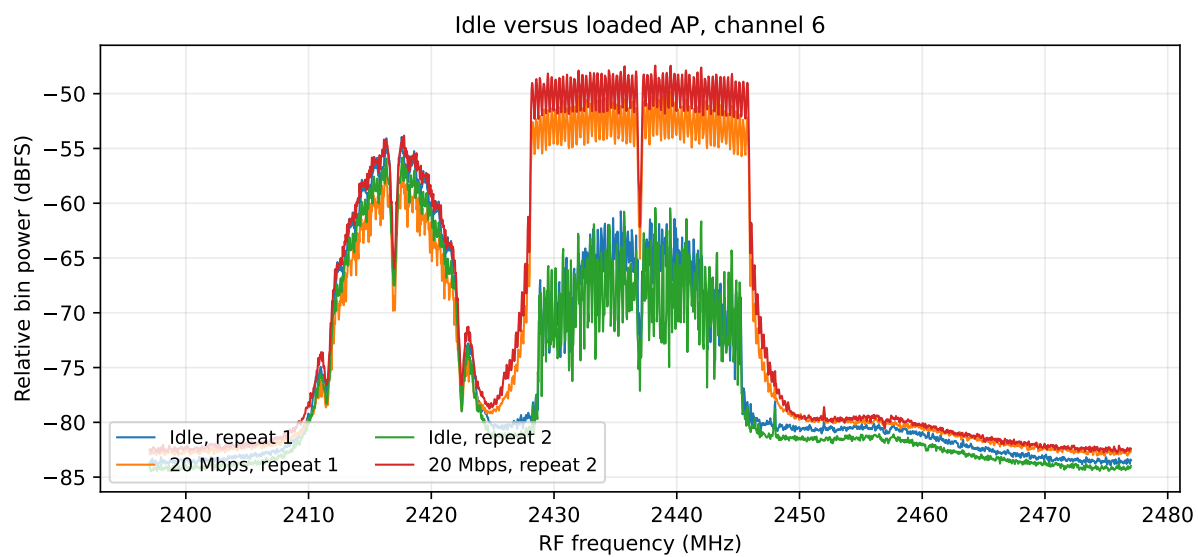
図 10 6 チャンネルの待機・負荷条件、各 2 回。少数の強い信号が線形平均へ寄与する。
