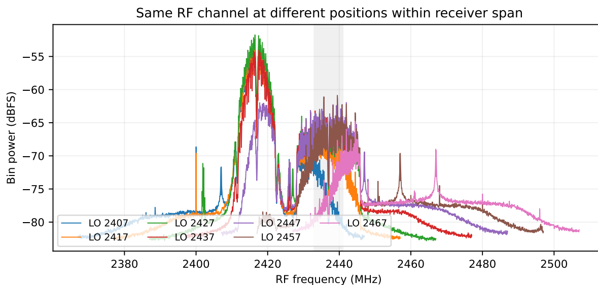
図 25 同一 RF チャンネルのスペクトルを LO 位置を変えて観測。灰色部分が比較用の固定 RF 帯域。
