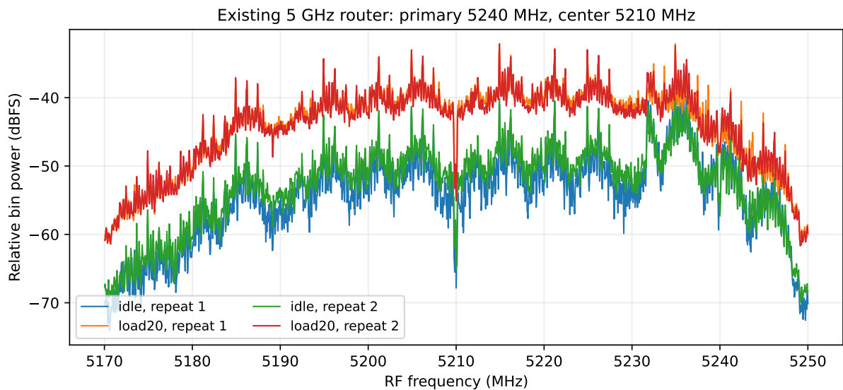
図 19 既存 5 GHz ルーターを用いた受信観測。BE200 が 5 GHz AP として動作した結果ではない。
