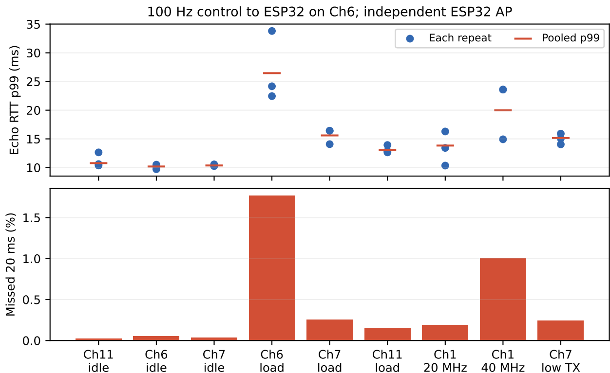
図 2 操縦側を Ch6 と ESP32-1 へ固定し、ESP32-2 AP の条件を変更した比較。idle は AP・ビーコンと TCP 接続を保ち、アプリの送信を止めた条件。load は TCP 飽和負荷で、等しい実効 Mbps を保証しない。
