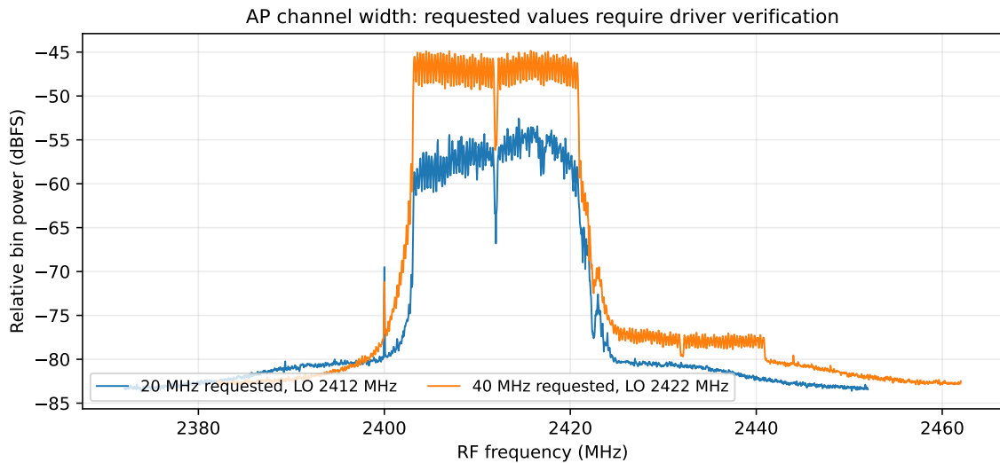
図 18 20 MHz 設定と 40 MHz 要求の比較。LO が異なるため、受信周波数応答の影響も含む。実際の帯域は結果表で確認する。
