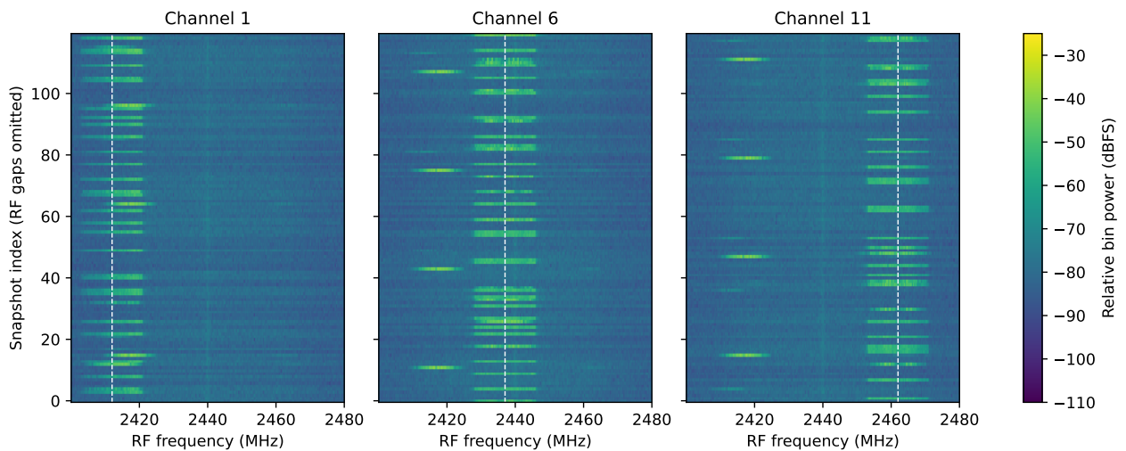
図 9 チャンネルごとの実測ウォーターフォール。破線は設定中心周波数。縦方向の隙間は未観測 RF 時間を表さず、取得番号を表す。
