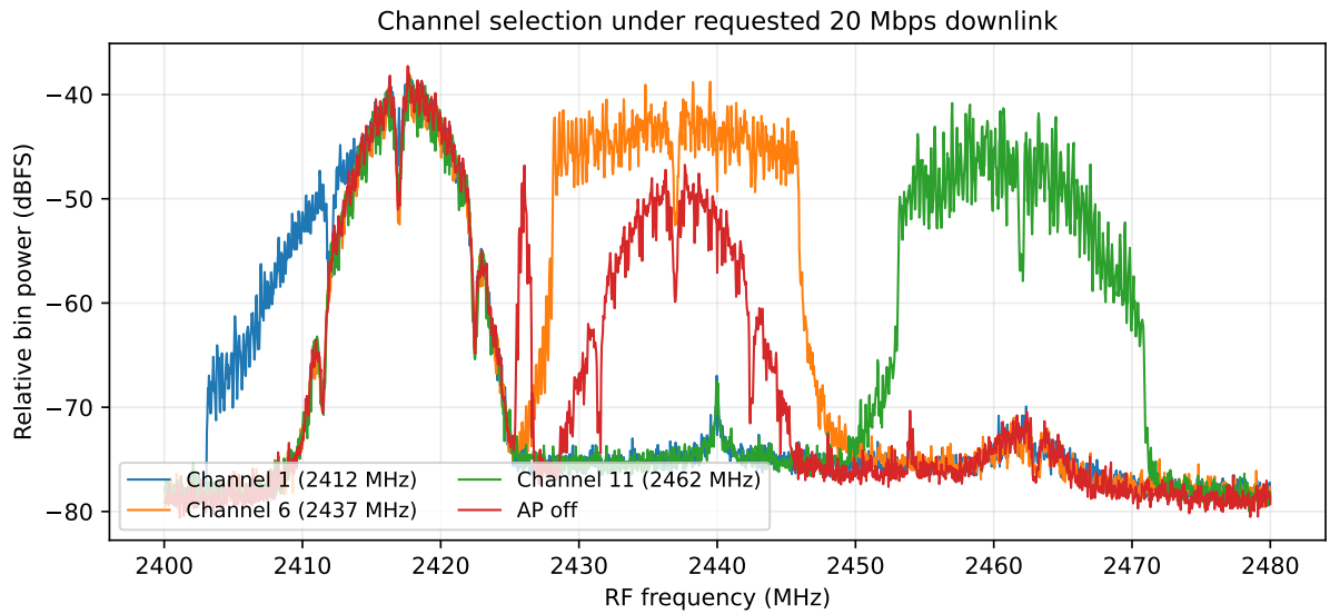
図 8 共通 LO=2440 MHz での最大スナップショット電力。設定チャンネルに対応する信号位置が変化する。AP 停止時にも外来信号がある。受信アナログ帯域の上限 48 MHz により 80 MHz 表示の端は同じ感度とは限らない。
