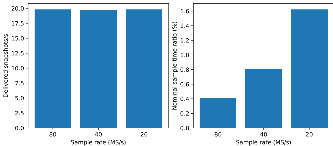
図 12 取得速度と名目サンプル時間比。全イベントを連続受信していると解釈しない。
