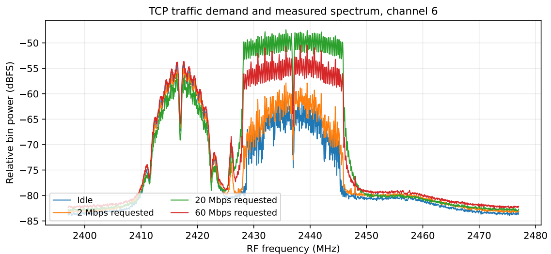
図 16 要求 TCP 速度 2・20・60 Mbps と待機条件。実効速度は結果表を参照。
