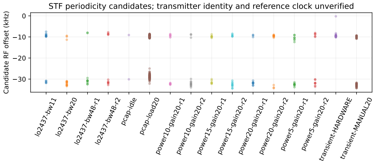
図 29 STF 周期性の条件を満たした周波数差候補。送信機の MAC 識別、RF 基準源、温度計測がないため、C5 の絶対周波数精度や温度ドリフトの校正値ではない。
