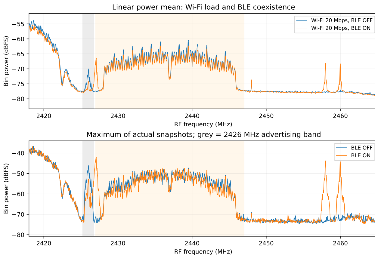
図 34 20 Mbps Wi-Fi 負荷と BLE の同時条件。両方とも実測であり、狭帯域成分の復号・送信機同定は行っていない。
