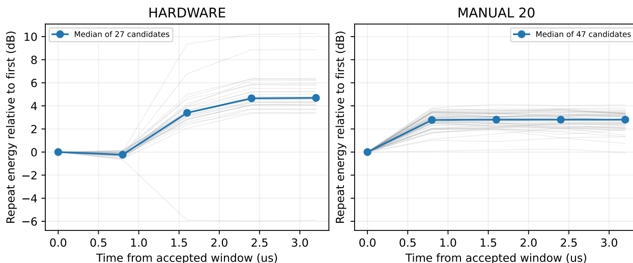
図 30 各 STF 候補の繰返しエネルギーを最初の受理周期で規格化。灰色は個別候補、太線は中央値。送信機混在、雑音、候補選択の影響を含む。
