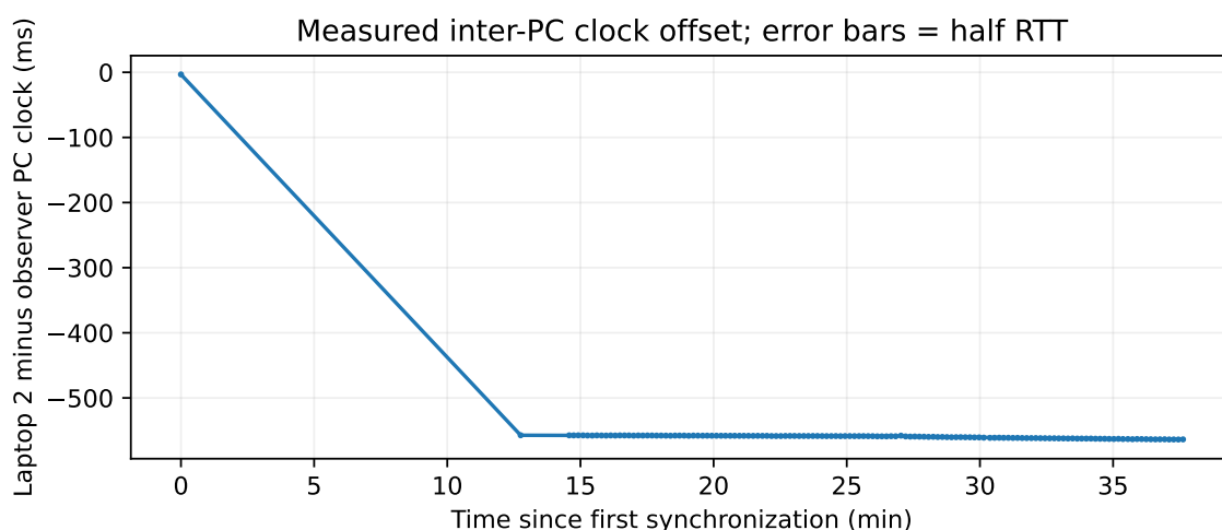
図 22 測定した PC 間時計差。誤差棒は半往復時間であり、スリープをまたぐ時計変化の上限ではない。
