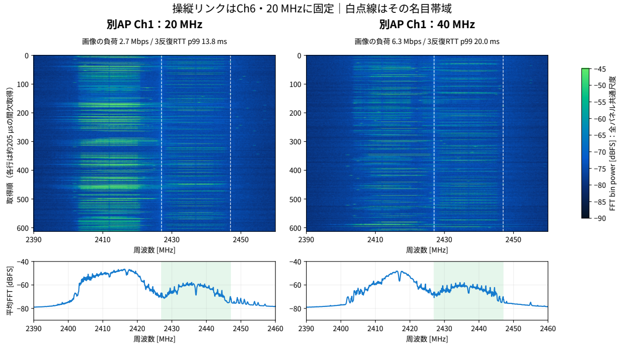
図5 Ch1 の 20/40 MHz 設定比較。同じ色尺度・LO=2427 MHz・ゲイン 20 で観察した。40 MHz の接続幅は 3 反復ともクライアントの iw ログで確認した。広い接続設定でも、全送信が 40 MHz 波形になるわけではなく、平均スペクトルを理想的な矩形に読み替えない。
