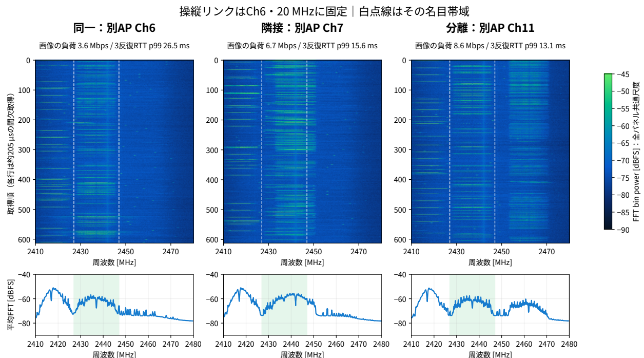
図4 青～緑の実測ウォーターフォール。画像は各条件の 1 反復目、RTT 注記は 3 反復の統合値。全パネルで同じ色尺度を使用し、白点線は操縦 Ch6 の名目範囲。2418 MHz 付近の強い成分など外来信号も含み、色を試験 AP だけに帰属しない。各行は約 205 \mu s の間欠取得であり、連続占有時間ではない。
