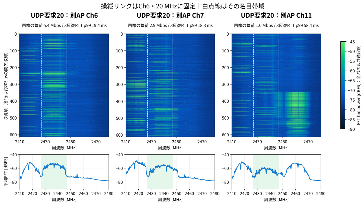
図 6 追加 UDP 要求 20 Mbps 条件の 1 反復目。色尺度は TCP 画像と同じ。要求値と実通信量が一致しないため、画面注記は実測受付量を使う。
