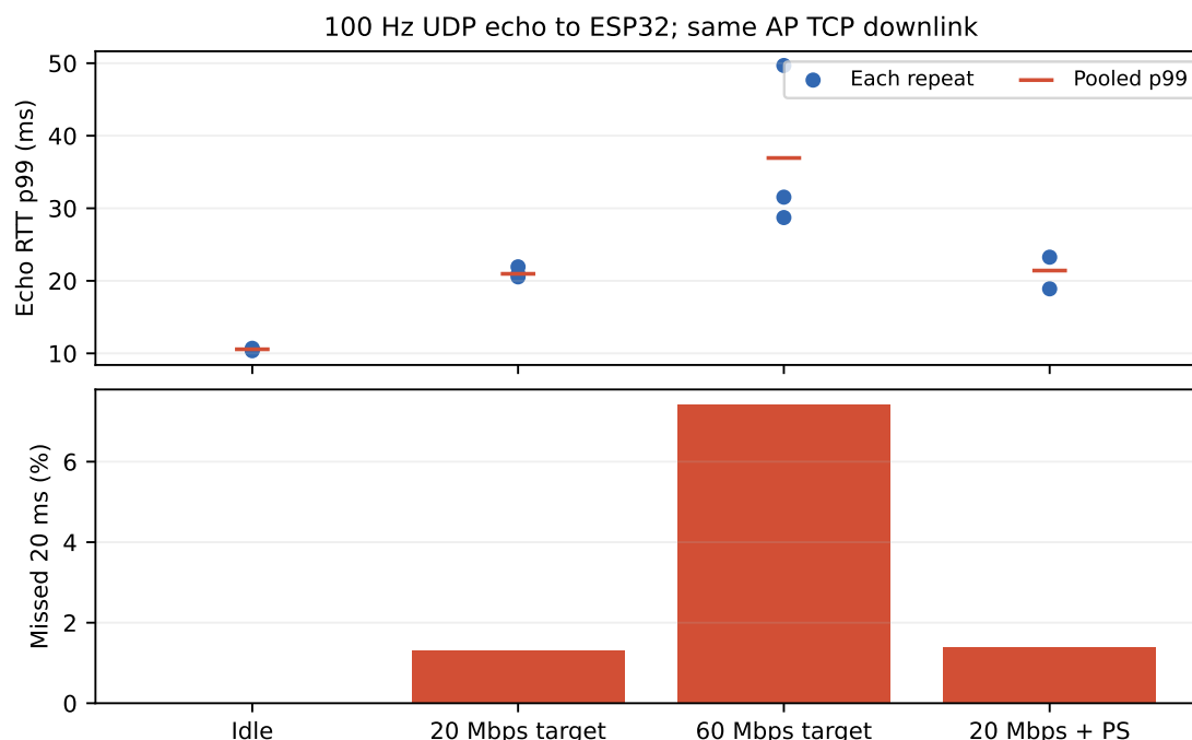
図 1 各反復の p99 と統合 p99、20 ms 期限超過率。負荷は TCP の指定値であり、60 Mbps 指定の実測は 38.4–40.6 Mbps であった。PS は ESP32 の Modem-sleep を有効にした補助比較。
