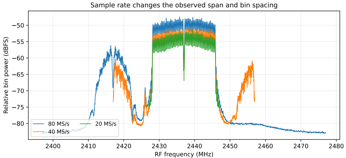
図 11 サンプルレート比較。同じ通信要求でも観測範囲とビン幅が変わる。
