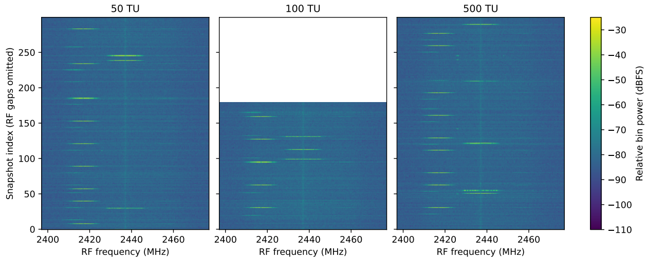
図 17 成功したビーコン設定の比較。短い取得と異なる取得回数のため、図の横縞の数だけで周期を比較しない。
