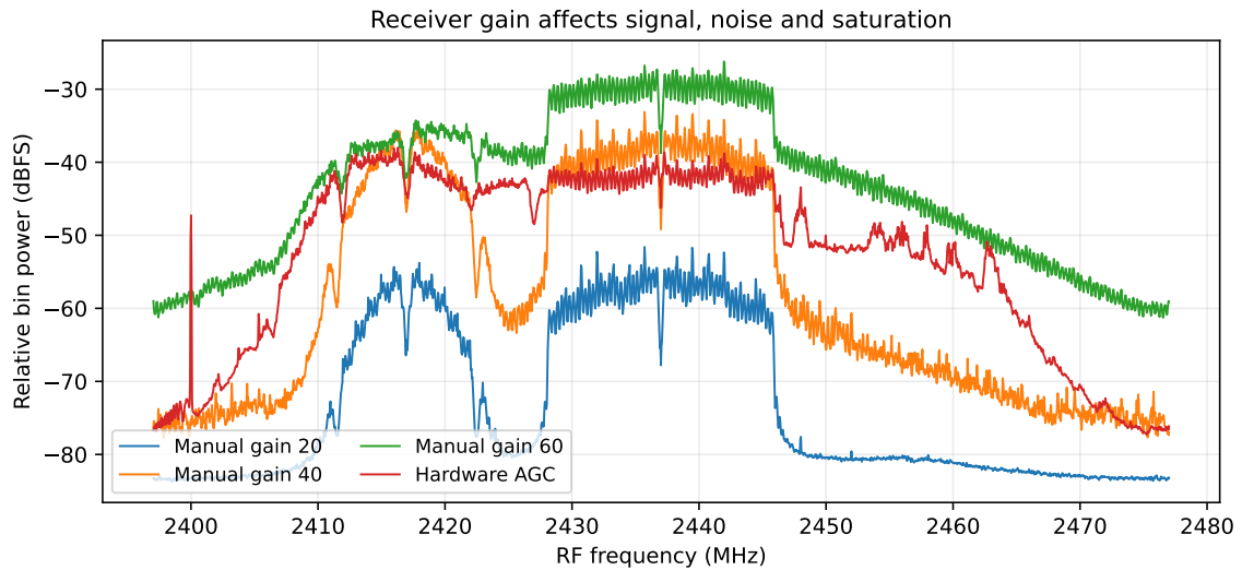
図 15 受信ゲインの比較。高い表示電力は受信感度や測定精度の改善を必ずしも意味しない。
