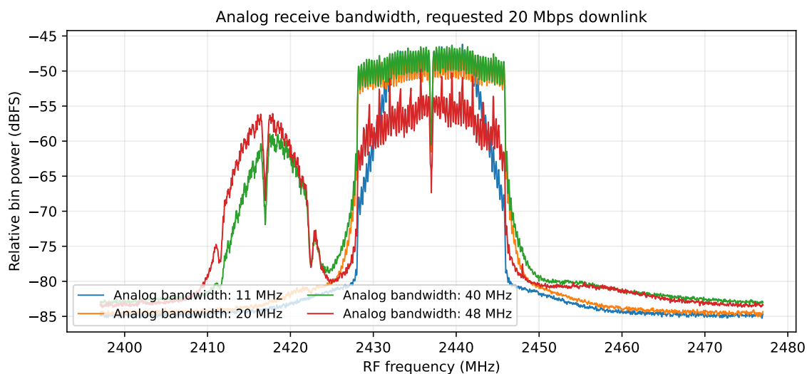
図 14 受信アナログ帯域の比較。表示スパンとアナログ通過帯域を区別する。
