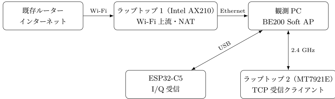
図 7 実験構成。制御は Tailscale SSH、負荷の TCP データは実験 AP のローカル IP 宛てに送る。C5 は周囲の信号も受信する。
