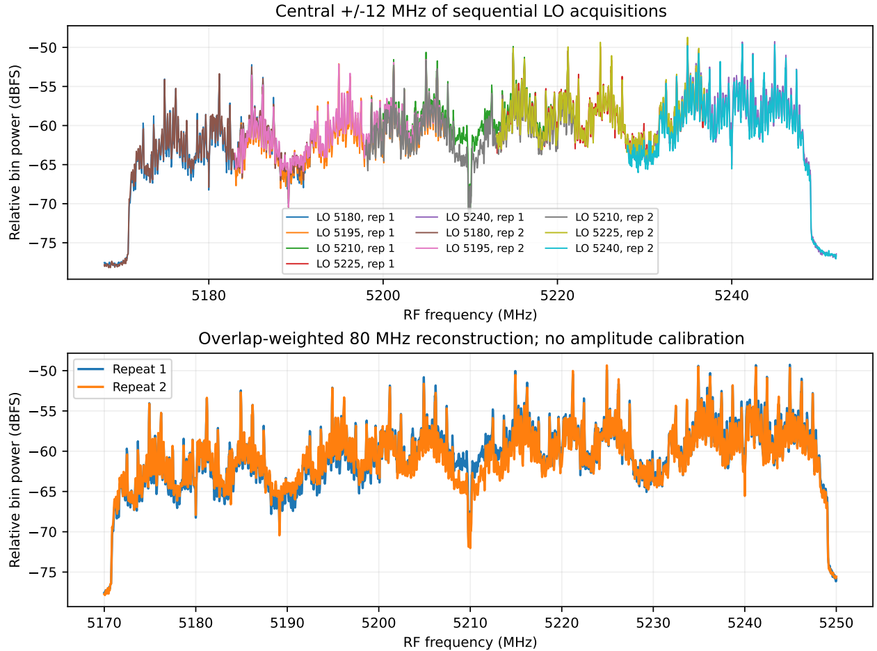
図 35 順次取得した中央スライスと 80 MHz 相当の重複合成。80 MHz を同時に連続受信した図ではなく、校正 PSD でもない。
