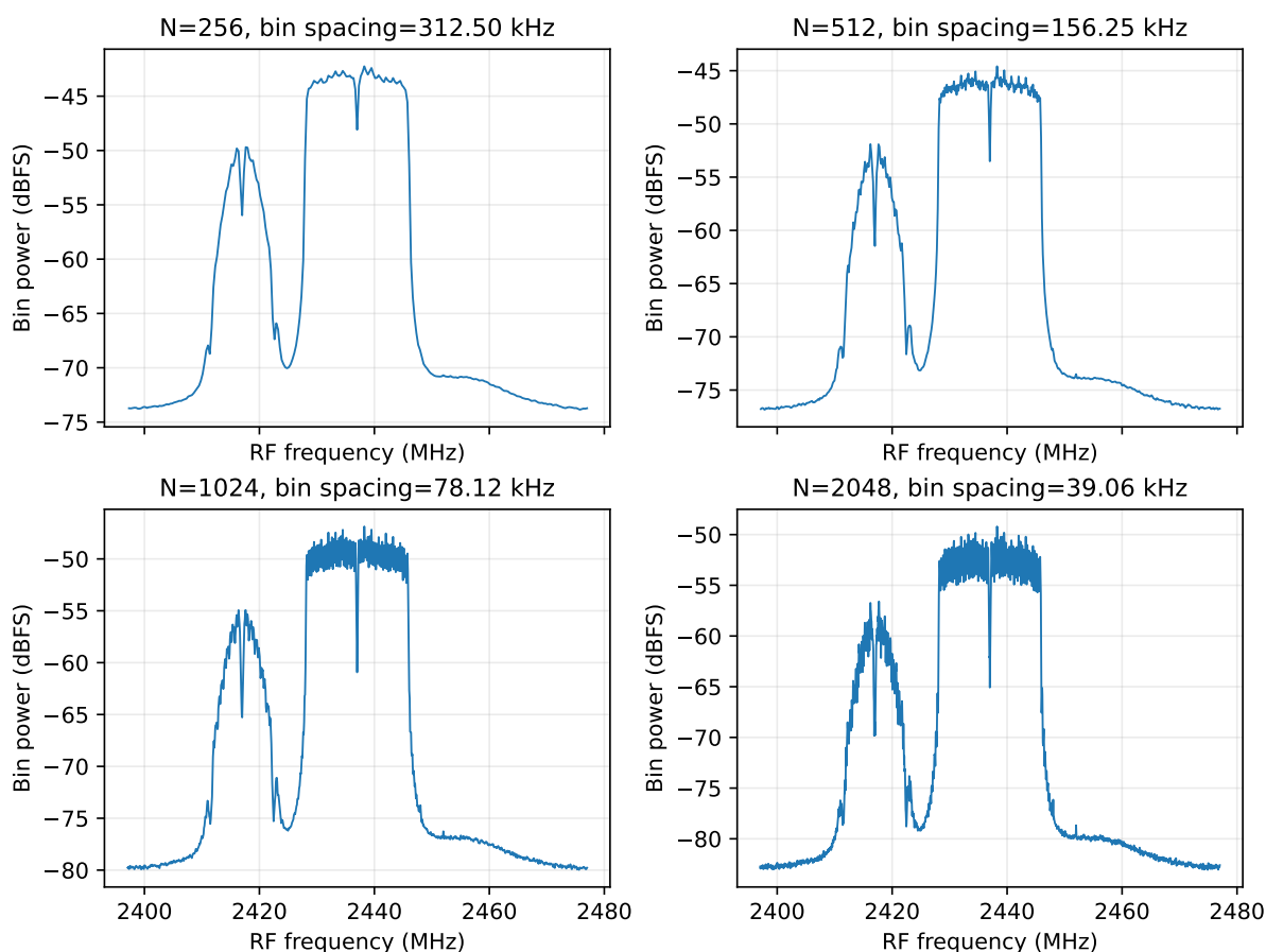
図 13 同一生データの FFT 長比較。ビン電力の規格化は同じだが、各ビンの帯域が異なる。
