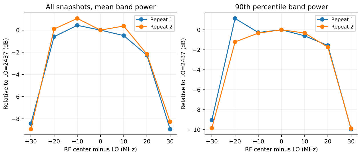
図 24 固定 RF 帯域の有効応答。各反復の中央 LO 条件を基準とする。縦軸は校正されたフロントエンド利得ではない。
