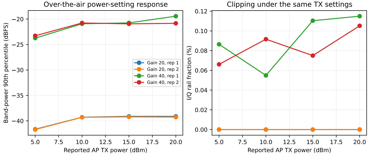
図 27 送信電力設定と受信帯域の 90 百分位・レール到達率。設定 dBm を C5 入力 dBm と置き換えない。
