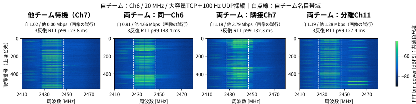
図 1: 他チームも通信中。同一・隣接・分離チャンネル、反復 1。青緑は未校正 dBFS、白線は名目帯域。
