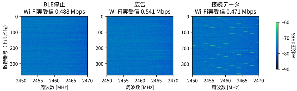
図 3: BLE 停止・広告・接続データ、Wi-Fi 負荷中・反復 1。2450–2470 MHz 拡大は広告 3 周波数と Wi-Fi Ch6 の名目帯域の外。
