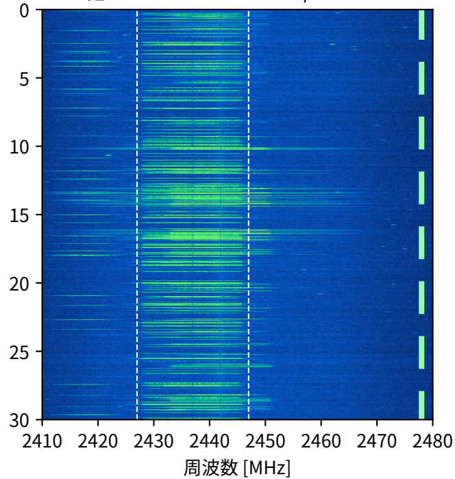
他チームCh7：2 s ON / 2 s OFF
