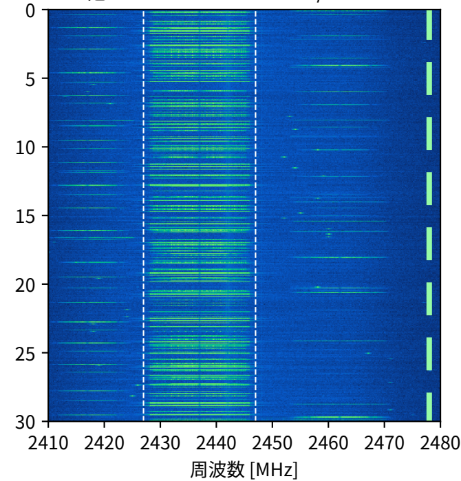
他チームCh11：2 s ON / 2 s OFF
