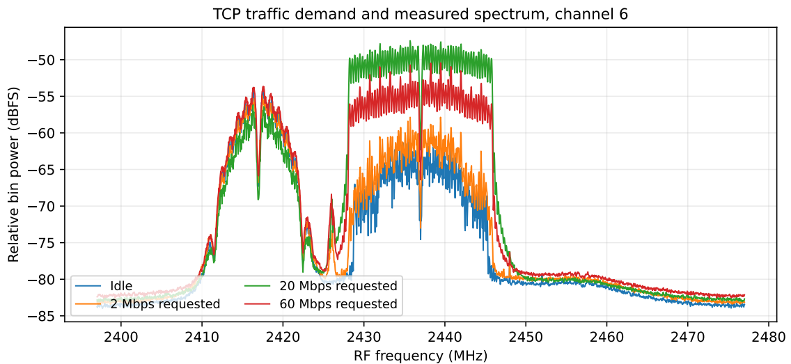
図 22: 要求 TCP 速度 2・20・60 Mbps と待機条件。実効速度は結果表を参照。
