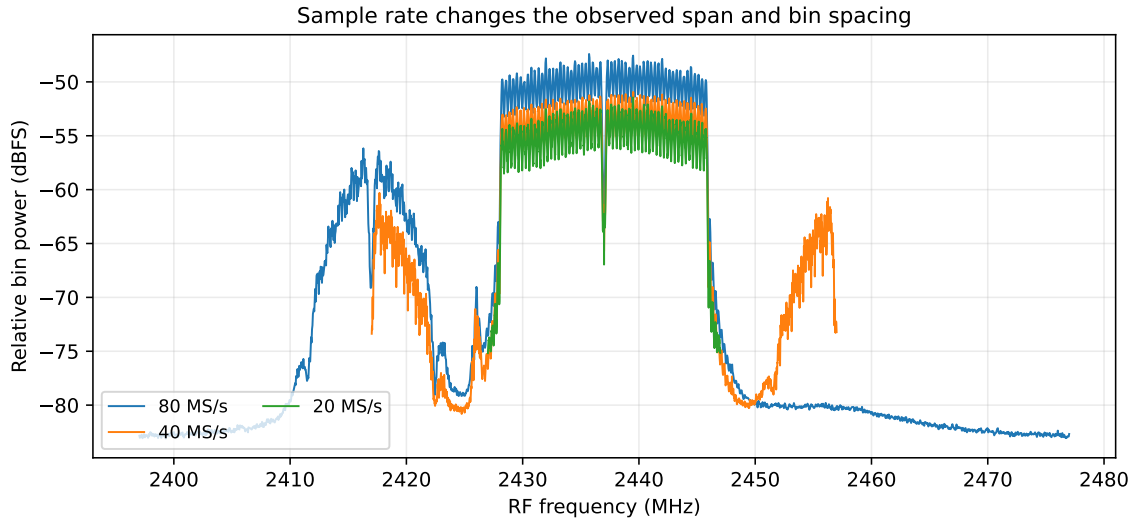
図 17: サンプルレート比較。同じ通信要求でも観測範囲とビン幅が変わる。
