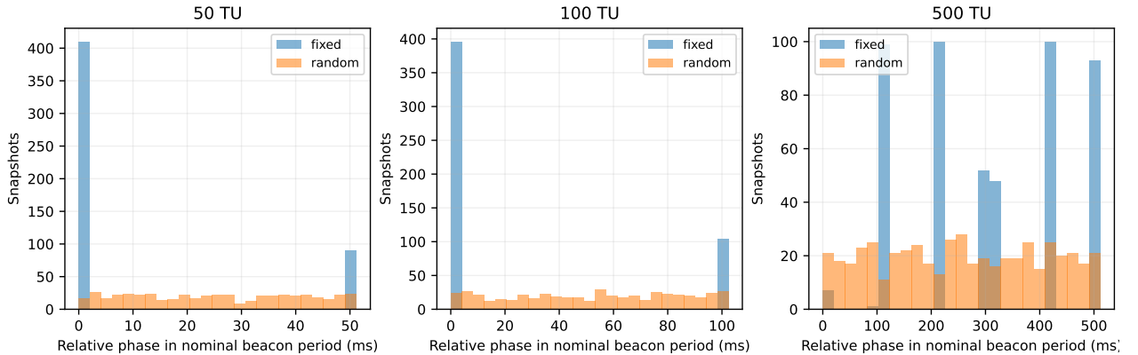
図 29: 名目ビーコン周期に対する取得位相。原点は各条件の最初の取得。絶対的なビーコン到着位相やパケット捕獲率の図ではない。
