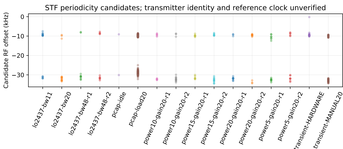
図 35: STF 周期性の条件を満たした周波数差候補。送信機の MAC 識別、RF 基準源、温度計測がないため、C5 の絶対周波数精度や温度ドリフトの校正値ではない。
