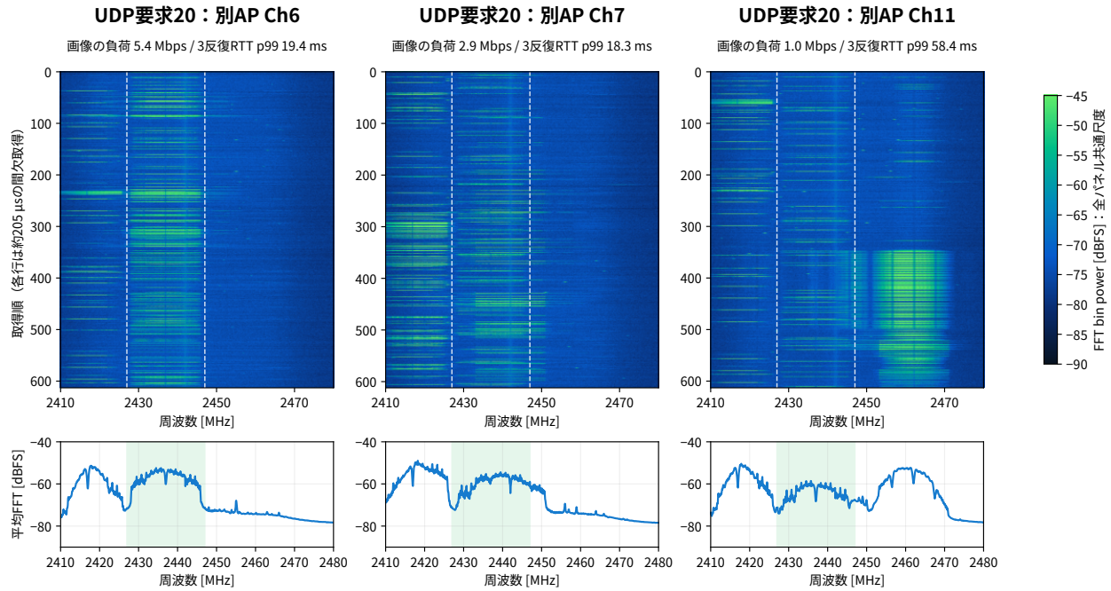
図 12: 追加 UDP 要求 20 Mbps 条件の 1 反復目。色尺度は TCP 画像と同じ。要求値と実通信量が一致しないため、画面注記は実測受付量を使う。
