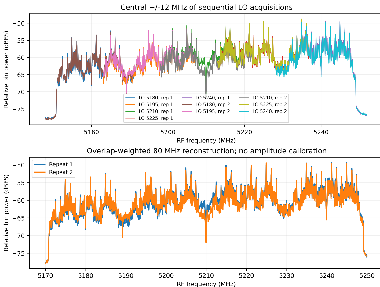
図 41: 順次取得した中央スライスと 80 MHz 相当の重複合成。80 MHz を同時に連続受信した図ではなく、校正 PSD でもない。
