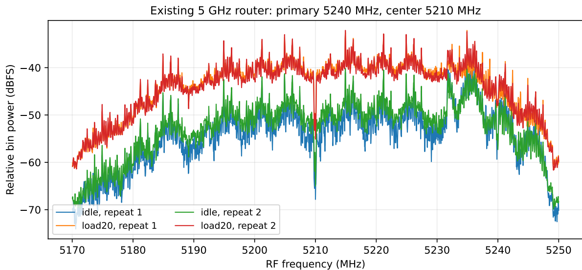
図 25: 既存 5 GHz ルーターを用いた受信観測。BE200 が 5 GHz AP として動作した結果ではない。
