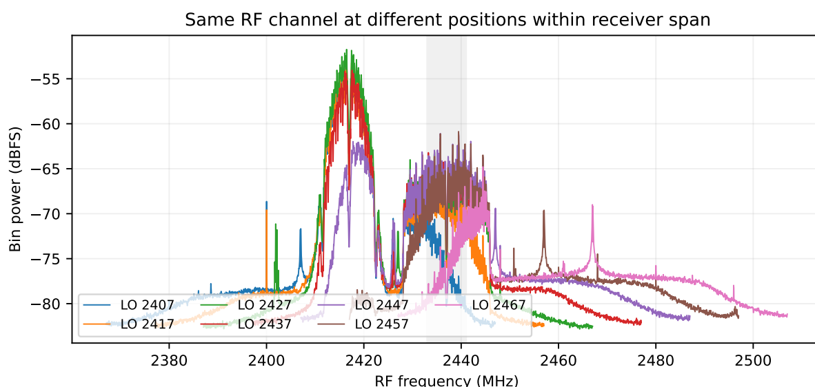
図 31: 同一 RF チャンネルのスペクトルを LO 位置を変えて観測。灰色部分が比較用の固定 RF 帯域。
