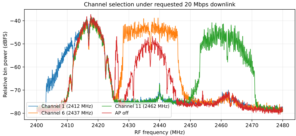
図 14: 共通 LO=2440 MHz での最大スナップショット電力。設定チャンネルに対応する信号位置が変化する。AP 停止時にも外来信号がある。受信アナログ帯域の上限 48 MHz により 80 MHz 表示の端は同じ感度とは限らない。
