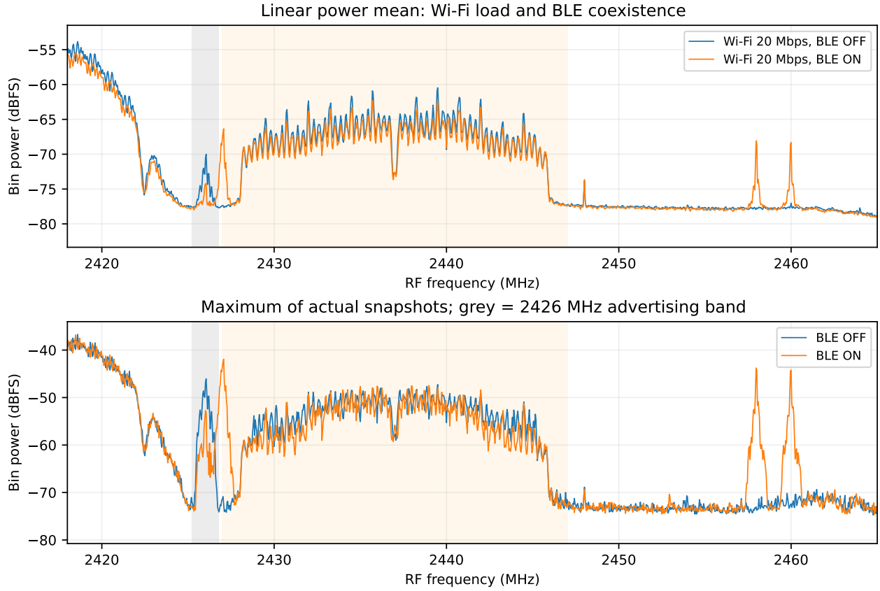
図 40: 20 Mbps Wi-Fi 負荷と BLE の同時条件。両方とも実測であり、狭帯域成分の復号・送信機同定は行っていない。
