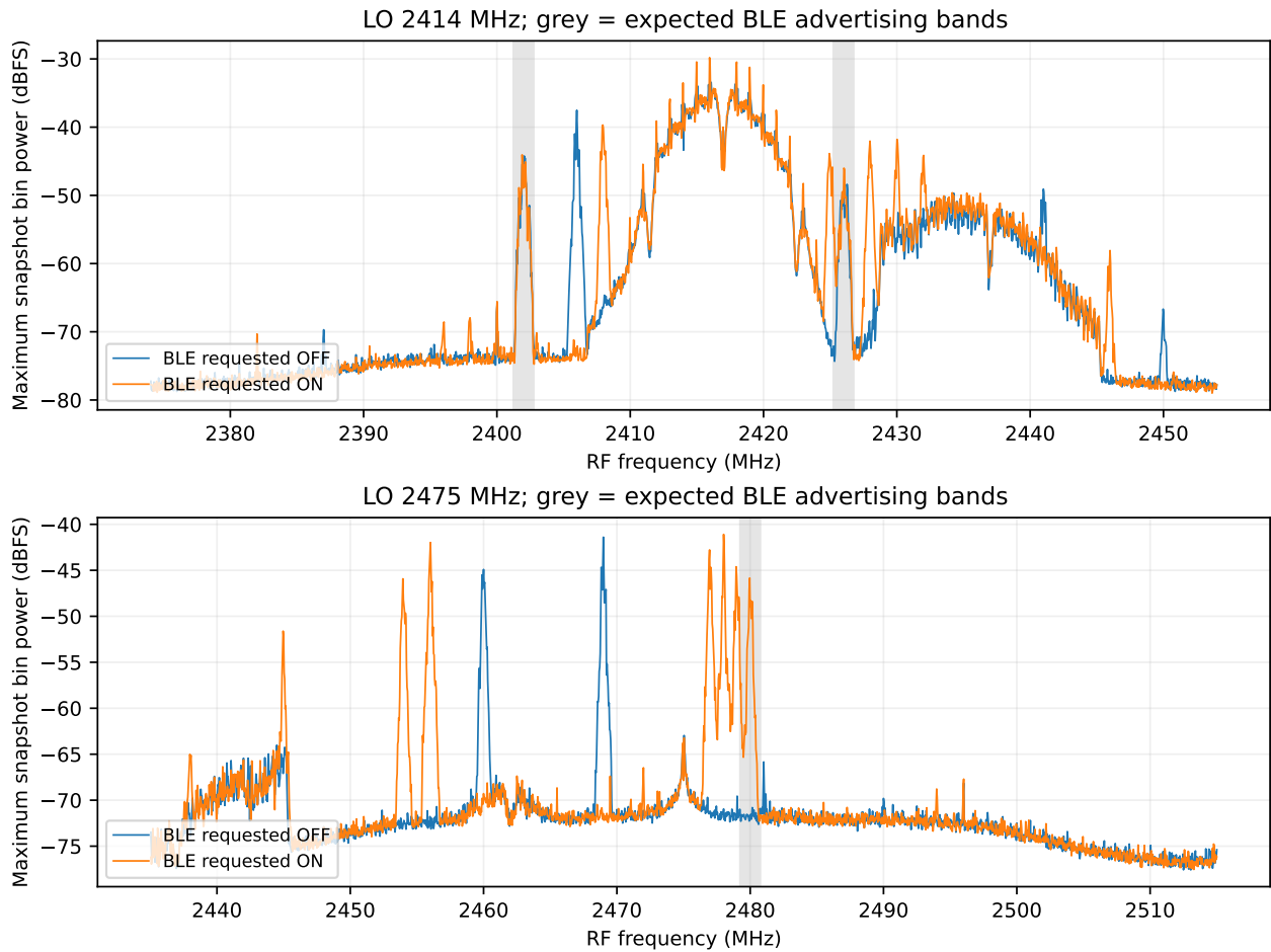
図 37: BLE ON/OFF の最大スナップショット電力。灰色は legacy 広告周波数付近。Wi-Fi 管理通信や他の Bluetooth 送信機も存在する。
