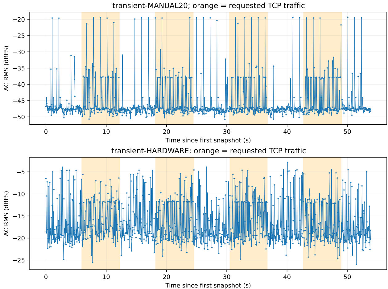
図 34: 全帯域 RMS の負荷過渡。橙色は TCP を要求した時間で、各パケットの実際の送信時刻ではない。
