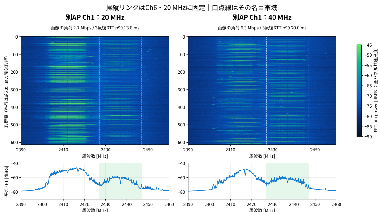
図 11: Ch1 の 20/40 MHz 設定比較。同じ色尺度・LO=2427 MHz・ゲイン 20 で観察した。40 MHz の接続幅は 3 反復ともクライアントの iw ログで確認した。広い接続設定でも、全送信が 40 MHz 波形になるわけではなく、平均スペクトルを理想的な矩形に読み替えない。
