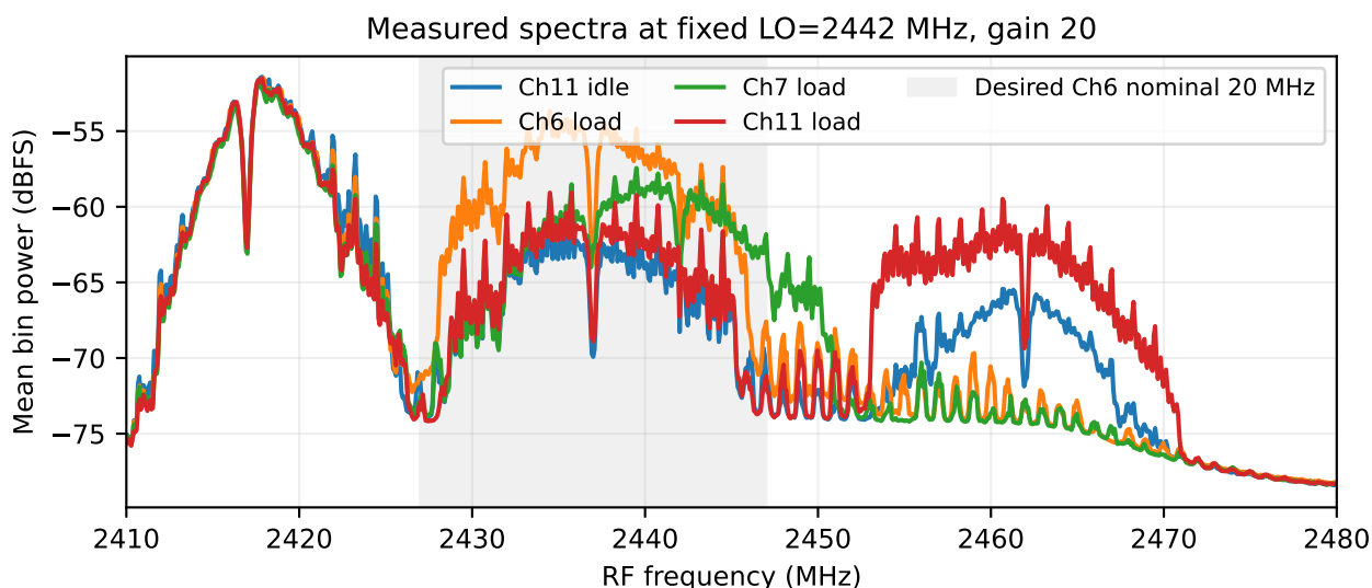
図 9: 独立 AP 比較の実測平均スペクトル。主 AP は Ch6 で固定。灰色は主 AP の名目 20 MHz 範囲。外来信号と受信機の周波数応答も含む。
