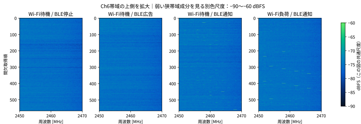
図 7: Ch6 の上側 2450–2470 MHz を拡大。弱い成分を読むため、この図内で共通の -90–-60 dBFS 尺度を使用する。前図とは同じ色が同じ電力を示さない。細線の全てを BLE へ帰属しない。
