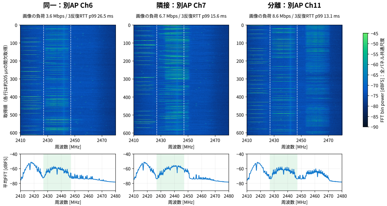
図 10: 青～緑の実測ウォーターホール。画像は各条件の 1 反復目、RTT 注記は 3 反復の統合値。全パネルで同じ色尺度を使用し、白点線は操縦 Ch6 の名目範囲。2418 MHz 付近の強い成分など外来信号も含み、色を試験 AP だけに帰属しない。各行は約 205 \mu s の間欠取得であり、連続占有時間ではない。
