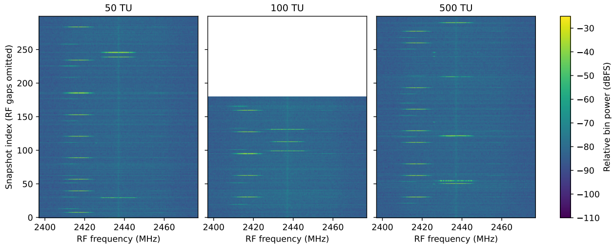
図 23: 成功したビーコン設定の比較。短い取得と異なる取得回数のため、図の横縞の数だけで周期を比較しない。
