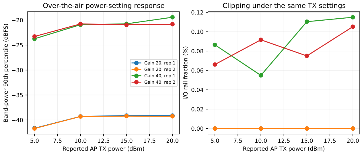
図 33: 送信電力設定と受信帯域の 90 百分位・レール到達率。設定 dBm を C5 入力 dBm と置き換えない。
