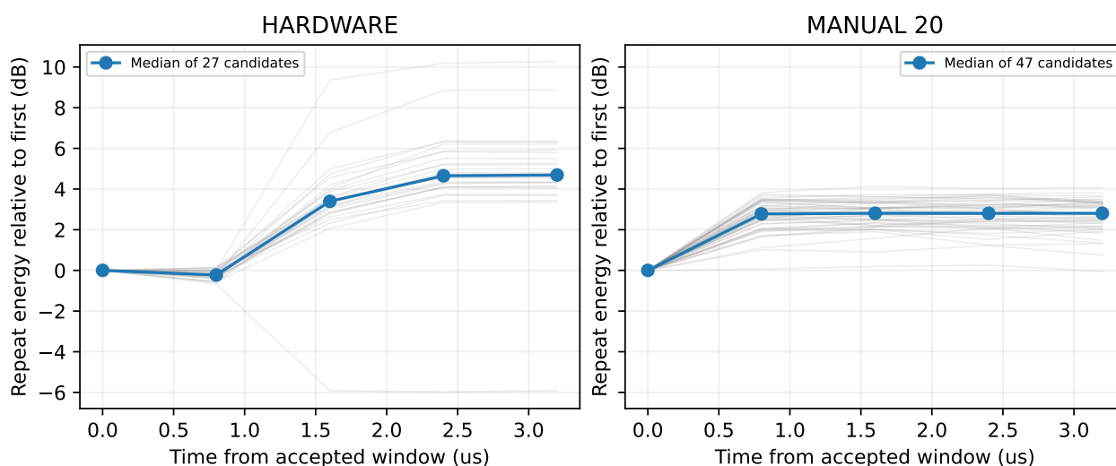
図 36: 各 STF 候補の繰返しエネルギーを最初の受理周期で規格化。灰色は個別候補、太線は中央値。送信機混在、雑音、候補選択の影響を含む。
