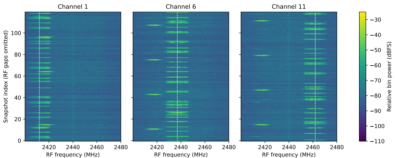
図 15: チャンネルごとの実測ウォーターフォール。破線は設定中心周波数。縦方向の隙間は未観測 RF 時間を表さず、取得番号を表す。
