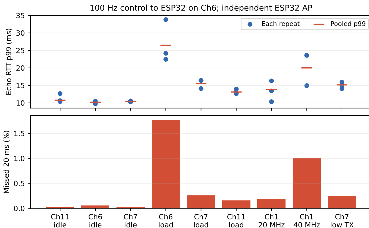
図 8: 操縦側を Ch6 と ESP32-1 へ固定し、ESP32-2 AP の条件を変更した比較。idle は AP・ビーコンと TCP 接続を保ち、アプリの送信を止めた条件。load は TCP 飽和負荷で、等しい実効 Mbps を保証しない。
