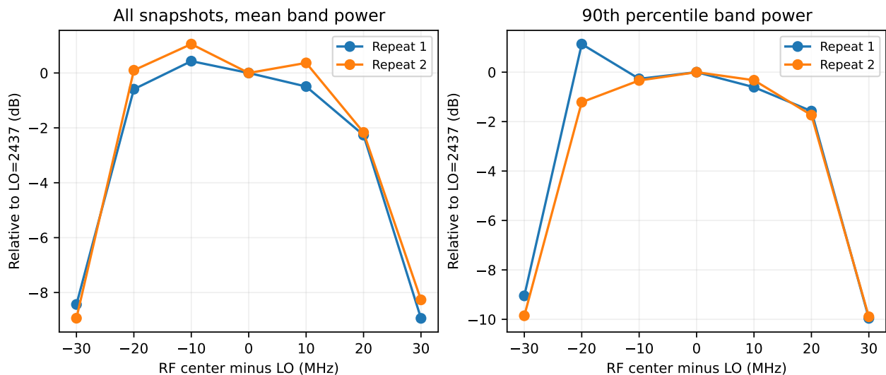
図 30: 固定 RF 帯域の有効応答。各反復の中央 LO 条件を基準とする。縦軸は校正されたフロントエンド利得ではない。
