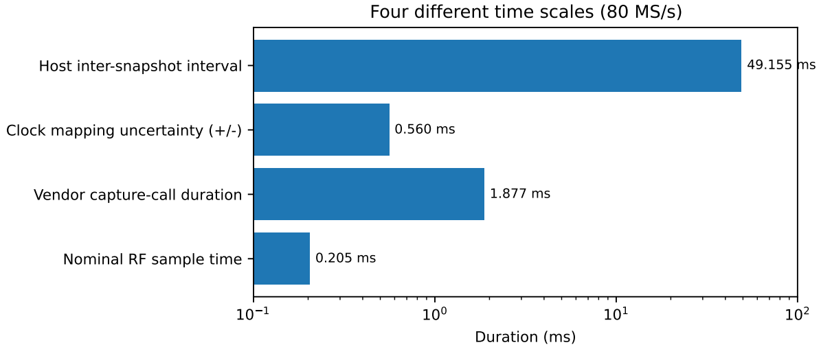
図 26: 別々の意味を持つ 4 種類の時間。対数軸。処理区間と名目 RF 時間を同一視しない。
