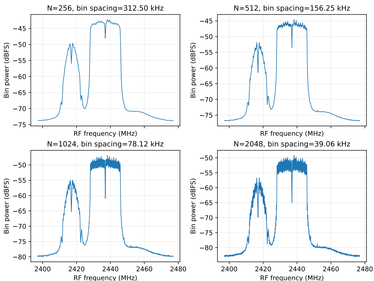
図 19: 同一生データの FFT 長比較。ビン電力の規格化は同じだが、各ビンの帯域が異なる。
