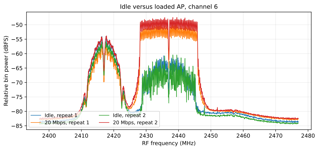
図 16: 6 チャンネルの待機・負荷条件、各 2 回。少数の強い信号が線形平均へ寄与する。
