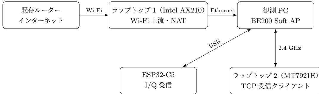
図 13: 実験構成。制御は Tailscale SSH、負荷の TCP データは実験 AP のローカル IP 宛てに送る。C5 は周囲の信号も受信する。
