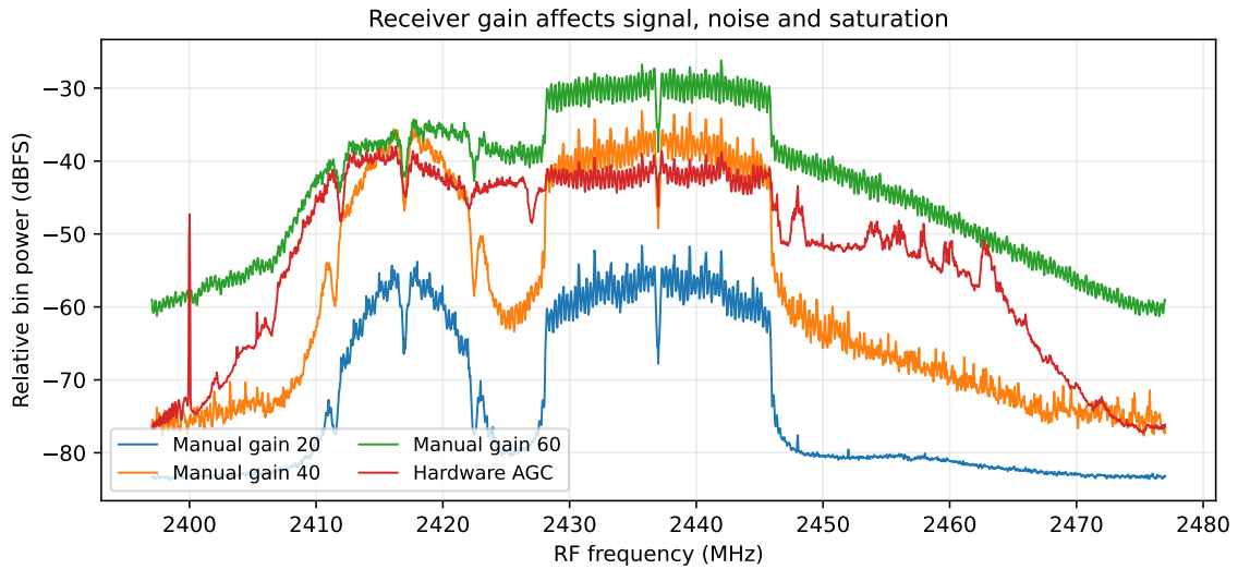
図 21: 受信ゲインの比較。高い表示電力は受信感度や測定精度の改善を必ずしも意味しない。
