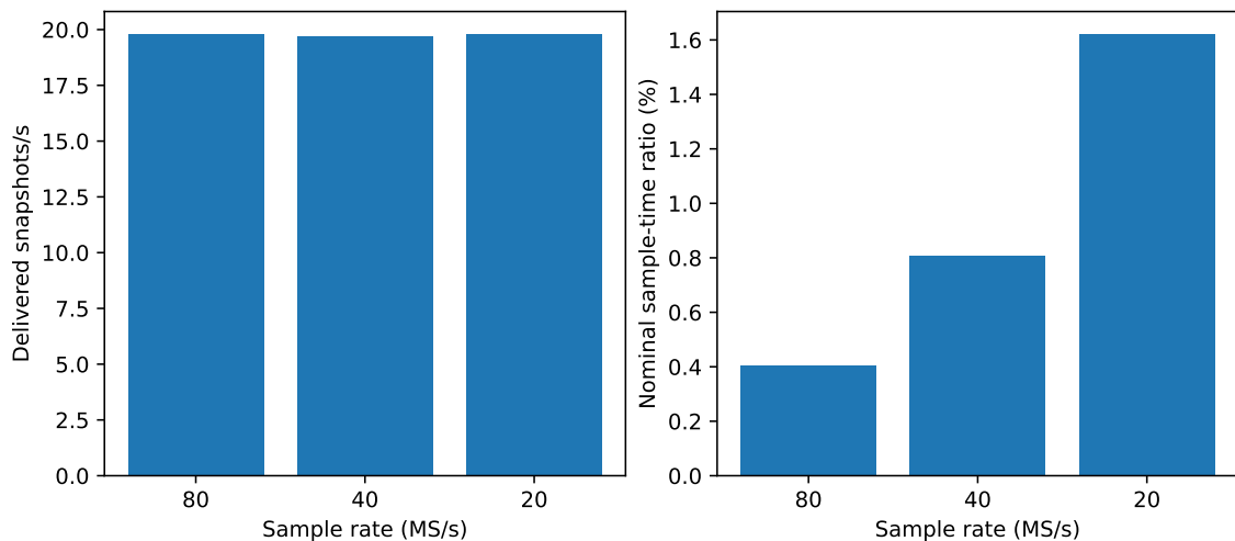
図 18: 取得速度と名目サンプル時間比。全イベントを連続受信していると解釈しない。
