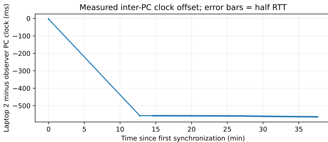
図 28: 測定した PC 間時計差。誤差棒は半往復時間であり、スリープをまたぐ時計変化の上限ではない。
