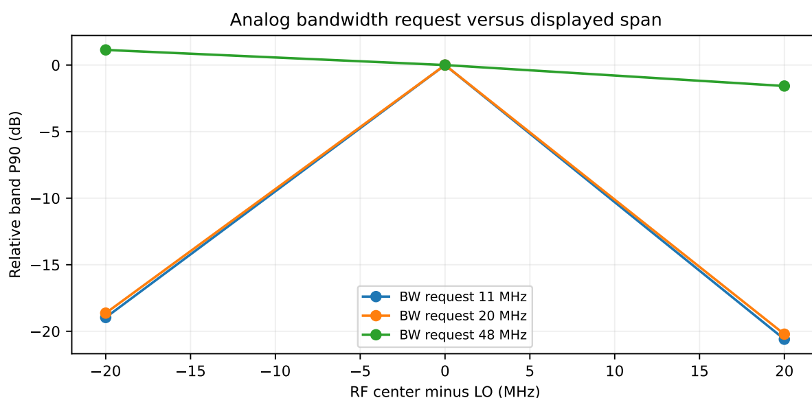
図 32: 11・20・48 MHz 帯域要求での固定 RF 帯域応答。48 MHz のみ 2 反復で、反復 1 を表示。各帯域の中央 LO 条件で規格化した。
