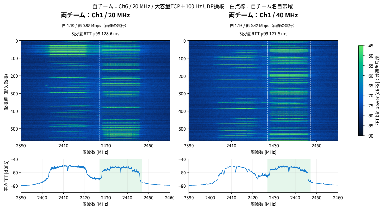
図 4: 他チーム Ch1 の 20/40 MHz。クライアントの接続幅と副チャネルを読み出した。
