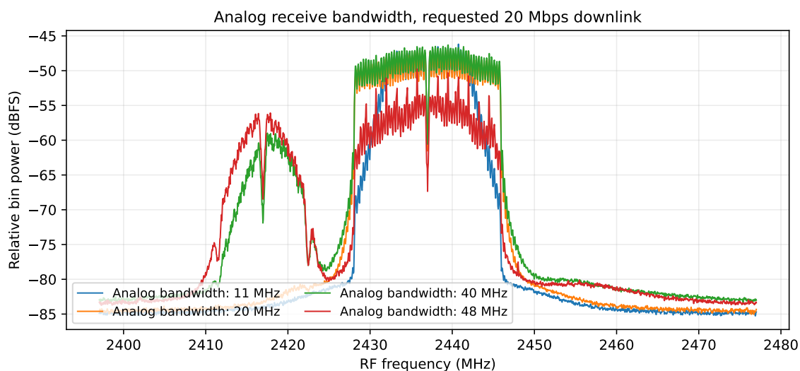
図 20: 受信アナログ帯域の比較。表示スパンとアナログ通過帯域を区別する。
