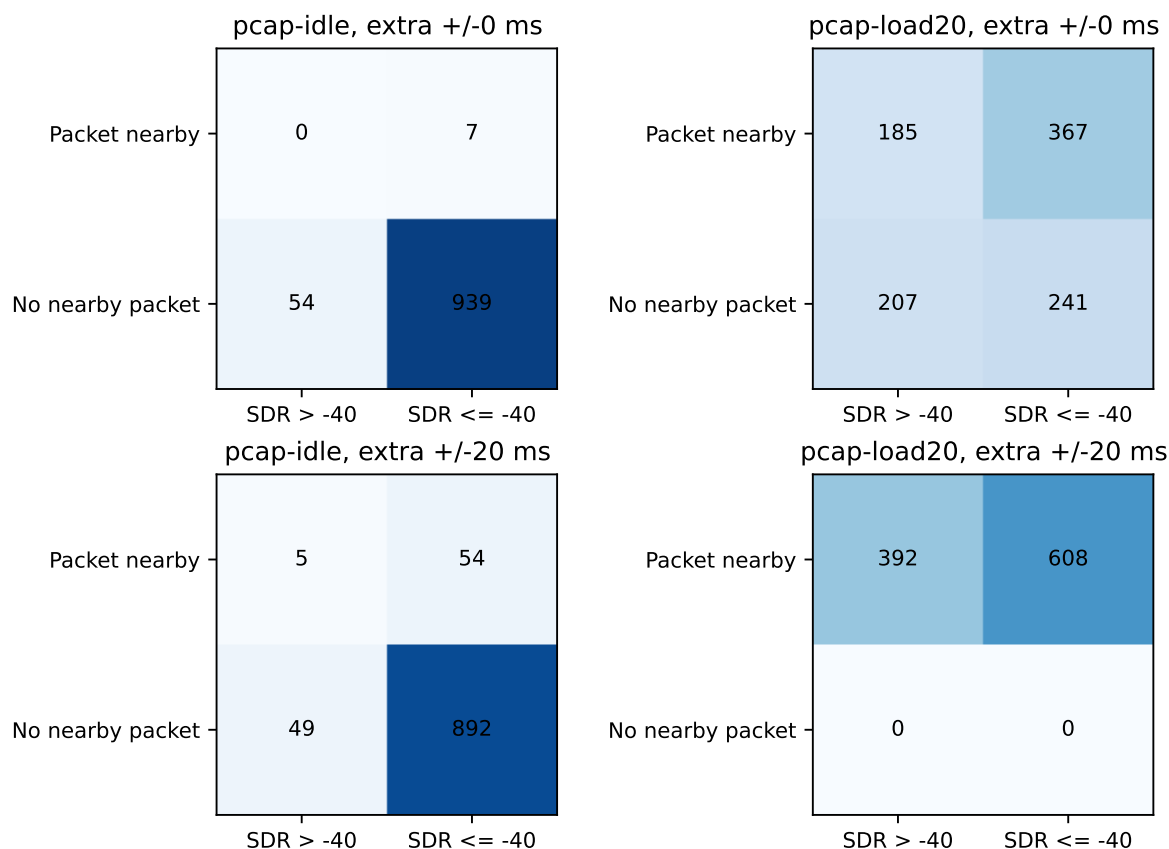
図 27: 時間窓を広げるだけでも関連表が変化する。送信通知を含む集計。ラベルを確定した検出器の混同行列ではない。
