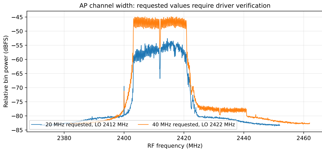
図 24: 20 MHz 設定と 40 MHz 要求の比較。LO が異なるため、受信周波数応答の影響も含む。実際の帯域は結果表で確認する。
