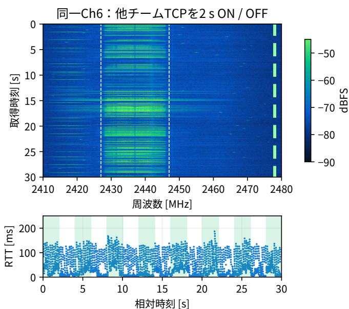
図 4: 上：実測 FFT。下：同じ試行の応答 RTT。緑帯は UART による ON 操作区間。両時計の対応は近似で、パケット単位の同期ではない。
