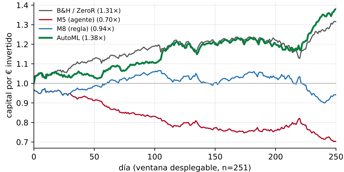
SPY: capital de las estrategias (AutoML supera a la trivial)
