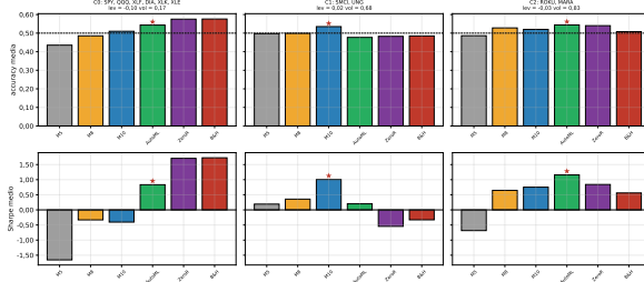
(a) Accuracy y Sharpe medios por estrategia dentro de cada grupo. Cada grupo se rescata por un canal distinto, coherente con su naturaleza.
