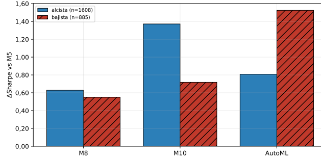
Figura 6.6: Complementariedad de los supervisores por régimen: \Delta\text{Sharpe} de M8, M10 y AutoML frente al agente, en mercado alcista y bajista. M10 rescata más en alcista, AutoML más en bajista; el contraste formal de ese reparto es la diferencia en diferencias ( \Delta\Delta\text{Sharpe} = +1,37 , p = 0,008 ).
