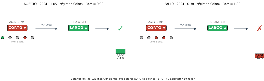
Figura 5.2: Anatomía de un día de intervención sobre SPY: la decisión del agente entra en RAM, que la compara con el régimen filtrado; si choca y el score supera \tau = 0,50 , la intervención la reorienta y el resultado se evalúa contra el retorno del día siguiente.
