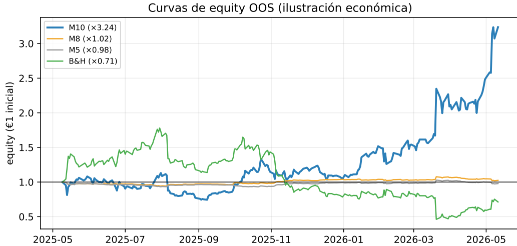
Figura 4.5: Curvas de capital sobre SMCI (OOS, n = 250 ): M10 (3,24×) frente a comprar-y-mantener (0,71×) y los demás baselines. Plano económico, ilustrativo. Fuente: notebooks/m10_better_smci.ipynb .
