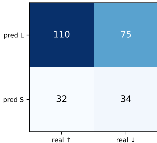
AutoML acc = 0,57
