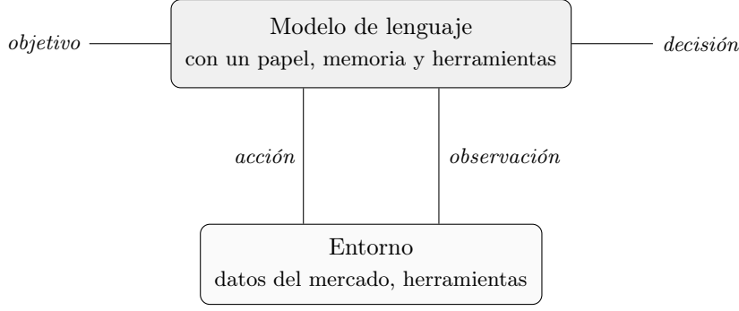
Figura 3.1: De modelo a agente. Un modelo de lenguaje aislado lleva una entrada a una salida en un solo paso. Un agente envuelve al modelo en un bucle: dotado de un papel, una memoria y unas herramientas, emite una acción sobre el entorno, observa el resultado y decide el paso siguiente, hasta una condición de parada que fija la decisión final. Esquema adaptado de Schluntz y Zhang [17].
