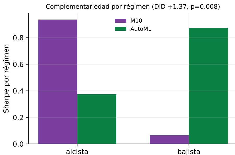
Figura 4.11: Complementariedad de los aprendices por régimen: \Delta\text{Sharpe} de M10 y de AutoML frente al agente, en alcista y en bajista. M10 rescata más en alcista, AutoML más en bajista; el contraste de diferencia-en-diferencias del reparto da \Delta\Delta\text{Sharpe} = +1,37 , \text{IC}_{95} [0,20, 2,60] , p = 0,008 (pooled; no significativo en SPY solo). Fuente: regime_did_learners.json .
