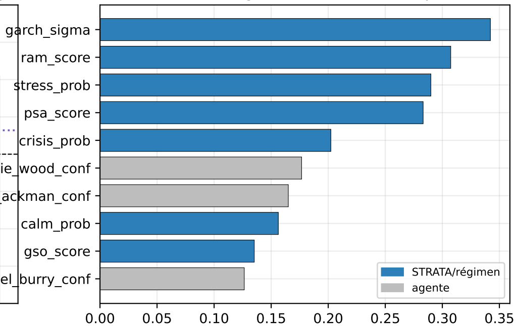
SHAP: STRATA/régimen = 65% de la importancia
