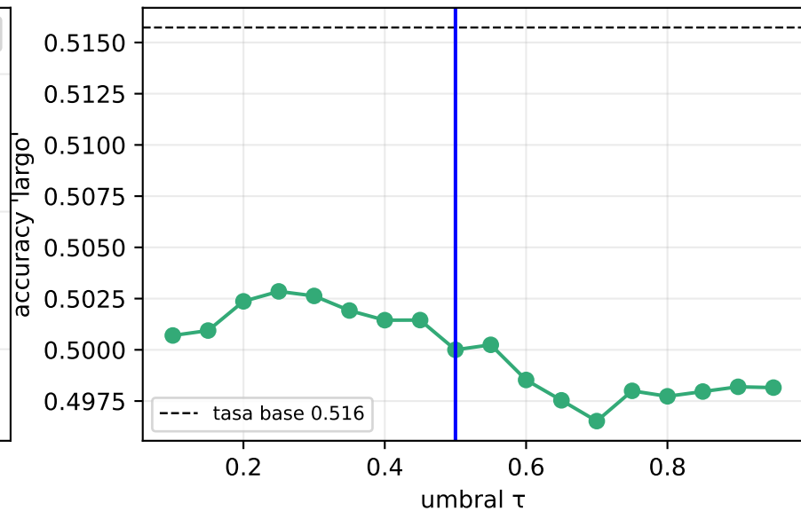
Accuracy plana \Rightarrow \tau no es un parámetro fino
