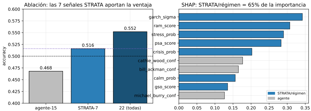
Figura 4.11: Izquierda: ablación (agente-15 \rightarrow 0,468, STRATA-7 \rightarrow 0,516, las 22 \rightarrow 0,552; McNemar 22 vs agente-15 p = 0,053 ). Derecha: importancia TreeSHAP, con las siete señales STRATA al 64,7 % y los cinco primeros features todas de STRATA y de régimen. Fuente: elaboración propia.
