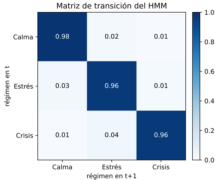
Figura 4.2: Matriz de transición del HMM sobre SMCI. La diagonal dominante refleja la persistencia de cada régimen (Calma \approx 45 días, Estrés \approx 25 , Crisis \approx 23 ). Fuente: elaboración propia.
