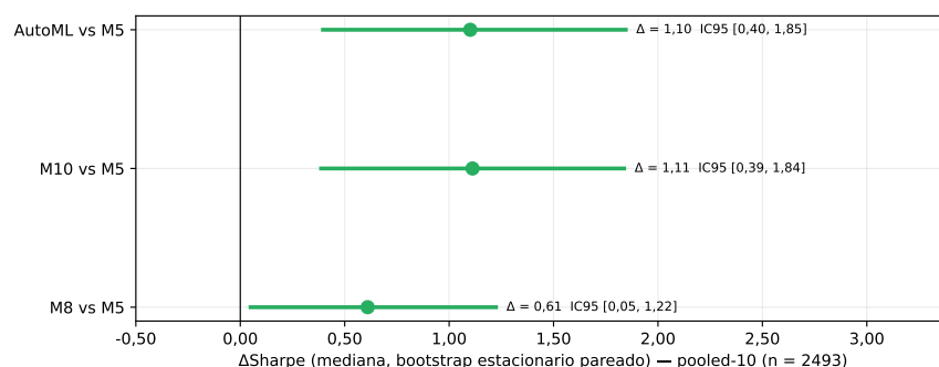
Figura 5.3: Diagrama de bosque del \Delta Sharpe pooled-10 frente al agente M5, con intervalo al 95 % ( bootstrap estacionario, Politis y Romano 1994). La línea vertical marca el cero. Los tres intervalos excluyen el cero; la regla M8 con el límite inferior más cerca del borde y los aprendices M10 y AutoML con más holgura. Fuente: bullbear_confirmatory.json (bloque POOLED10).
