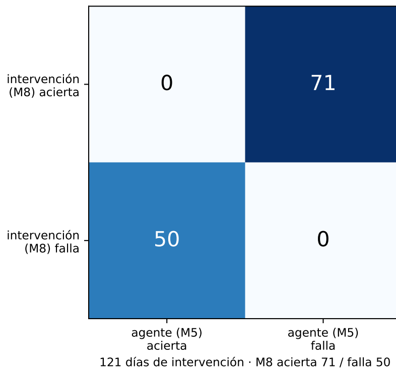
Figura 4.3: Matriz de confusión de la intervención sobre SPY: dirección del agente (M5) frente a dirección tras intervenir (M8), sobre las 121 intervenciones. La diagonal de rescate (71 aciertos de la intervención cuando el agente fallaba) supera a la de daño (50). Fuente: spy_intervention_anatomy.json .
