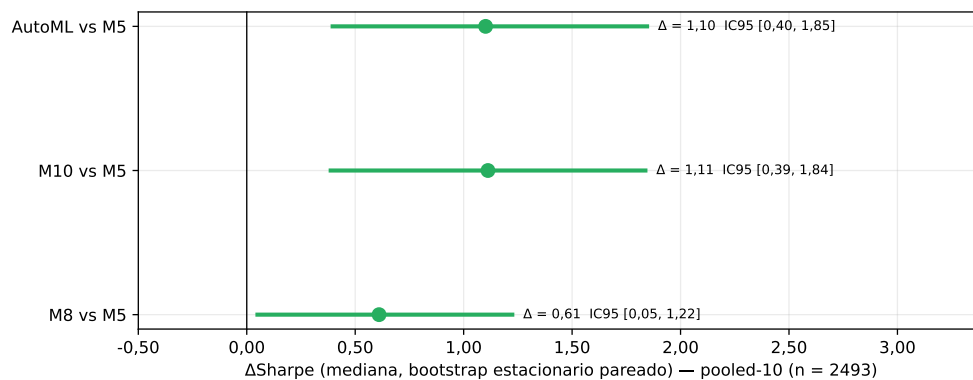
Figura 4.8: Diagrama de bosque del \Delta\text{Sharpe} pooled-10 frente al agente M5, con intervalo al 95 % ( bootstrap estacionario, Politis y Romano 1994) y cota inferior corregida por Bonferroni ( m = 3 ). La línea vertical marca el cero. Los tres intervalos simples excluyen el cero; bajo Bonferroni, M10 y AutoML se mantienen positivos y M8 toca el cero (cota inferior −0,047). Fuente: bullbear_confirmatory.json (bloque POOLED10).
