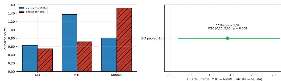
Figura 4.11: Complementariedad de los aprendices por régimen: \Delta\text{Sharpe} de M10 y de AutoML frente al agente, en alcista y en bajista. M10 rescata más en alcista, AutoML más en bajista; el contraste de diferencia-en-diferencias del reparto da \Delta\Delta\text{Sharpe} = +1,37 , \text{IC}_{95} [0,20, 2,60], p = 0,008 (pooled; no significativo en SPY solo). Fuente: regime_did_learners.json .
