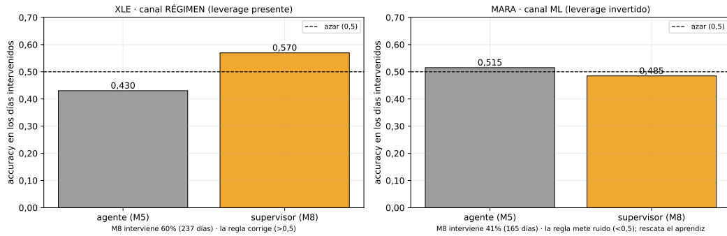
Figura 4.15: Dos casos trabajados, uno por canal. A la izquierda, XLE ( leverage fuerte): el régimen es direccional y la regla rescata el riesgo del agente. A la derecha, MARA ( leverage invertido): el régimen no informa el signo y el aprendiz rescata por la vía del sesgo del agente cruzado con el régimen. Cada panel muestra la dirección del agente, la del supervisor que rescata y el régimen vigente. Fuente: cluster_panel10.json , mechanism_panel.json .
