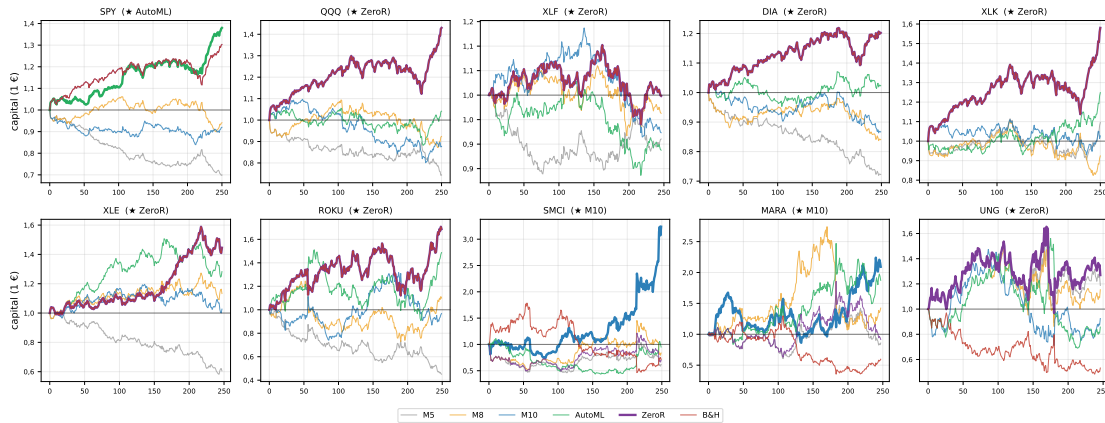
Figura 4.9: Curvas de capital por activo (un euro inicial), con la mejor derivada de STRATA destacada frente a las referencias. En cuatro activos una derivada bate al pasivo en Sharpe: SPY, SMCI, MARA y UNG. En SMCI/MARA/UNG el pasivo pierde o ronda el cero y la derivada saca Sharpe positivo yendo defensiva (lectura de valor direccional); en SPY la ventaja es sobre todo beta de mercado en un periodo alcista. Lectura sin contraste asociado. Fuente: automl_net_returns.json .
