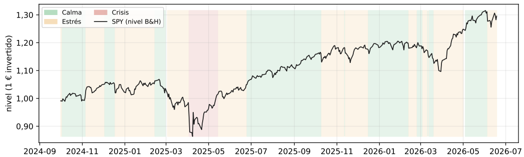
Figura 4.1: Regímenes del HMM ( K = 3 ) sobre el precio de SPY en el periodo de evaluación. Calma (volatilidad baja, retorno medio positivo), Estrés (intermedio) y Crisis (volatilidad alta, retorno medio negativo) ordenan por la firma del leverage effect . El sombreado marca el régimen vigente cada día; la coincidencia régimen \leftrightarrow caída es contemporánea, no predictiva. Fuente: regime_direction_table.json .
