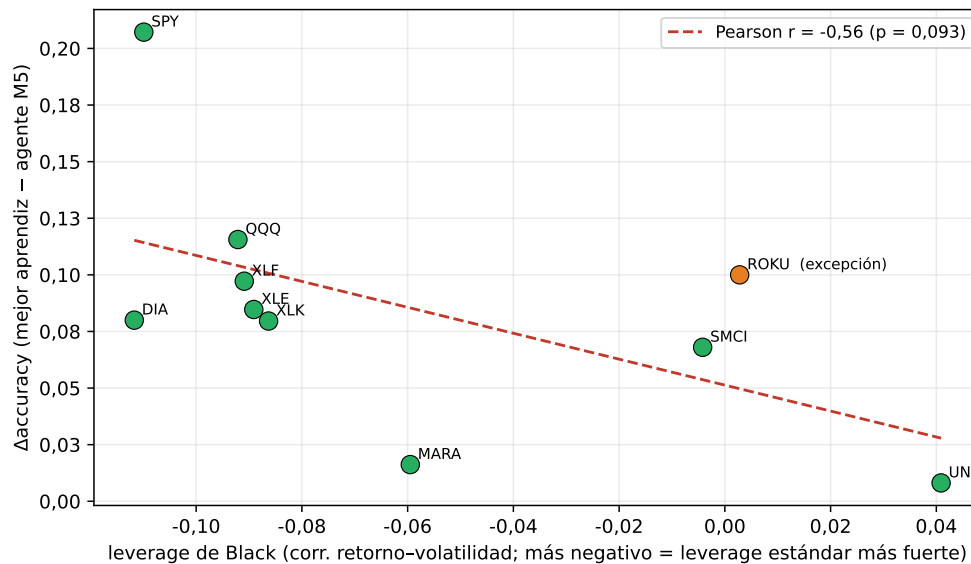
Figura 4.13: Rescate del aprendiz en accuracy frente al leverage del activo, sobre los diez. Cada punto es un activo; el eje horizontal es la correlación de Black \text{corr}(r_t, \text{RV}_{t+1}^{21} - \text{RV}_t^{21}) , el vertical el rescate \max(\text{M10}, \text{AutoML}) - \text{M5} . La recta de regresión baja con el leverage : a más leverage negativo, más rescate (Pearson r = -0,56 , p = 0,093 ; tendencia significativa al \alpha = 0,10 pre-registrado). Nueve de los diez la siguen; ROKU, señalado, es la excepción. Fuente: leverage_law_panel10.json .
