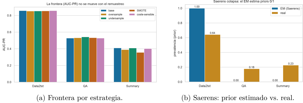
Figura 1.18: Reequilibrar clases no mueve la frontera; la corrección de prior de Saerens colapsa. Resultados negativos, documentados por honestidad.
