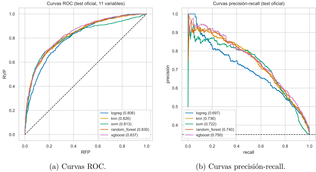
Figura 1.13: Discriminación de los cinco modelos sobre el test oficial (once variables).
