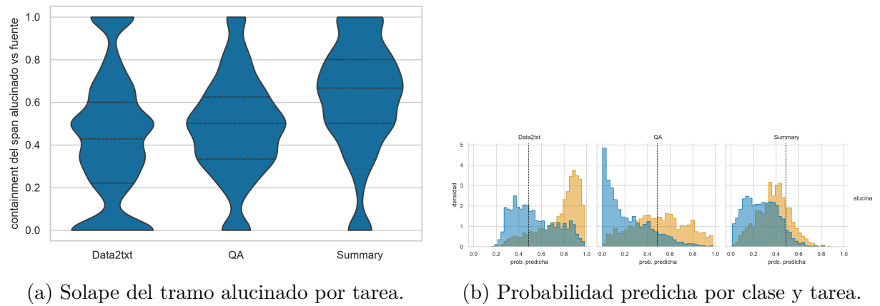
Figura 1.19: El cuello de botella de Summary es el camuflaje léxico, no el tipo de alucinación.
