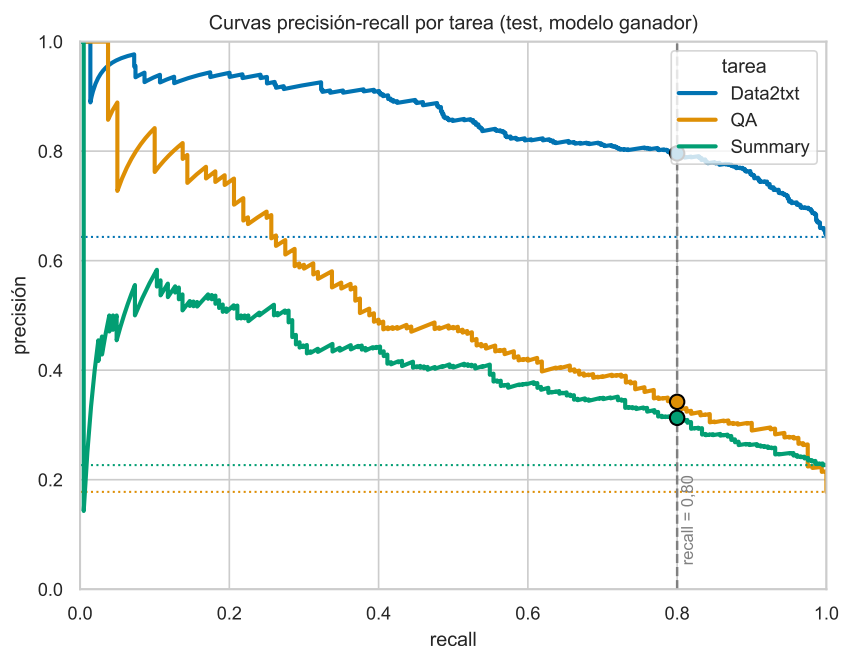
Figura 1.14: Curvas precisión-recall por tarea con la línea base en y = \text{prevalencia} . Fijar un recall del 80% cuesta poca precisión en Data2txt y mucha en Summary: ese es el compromiso rigor–precisión del detector.
