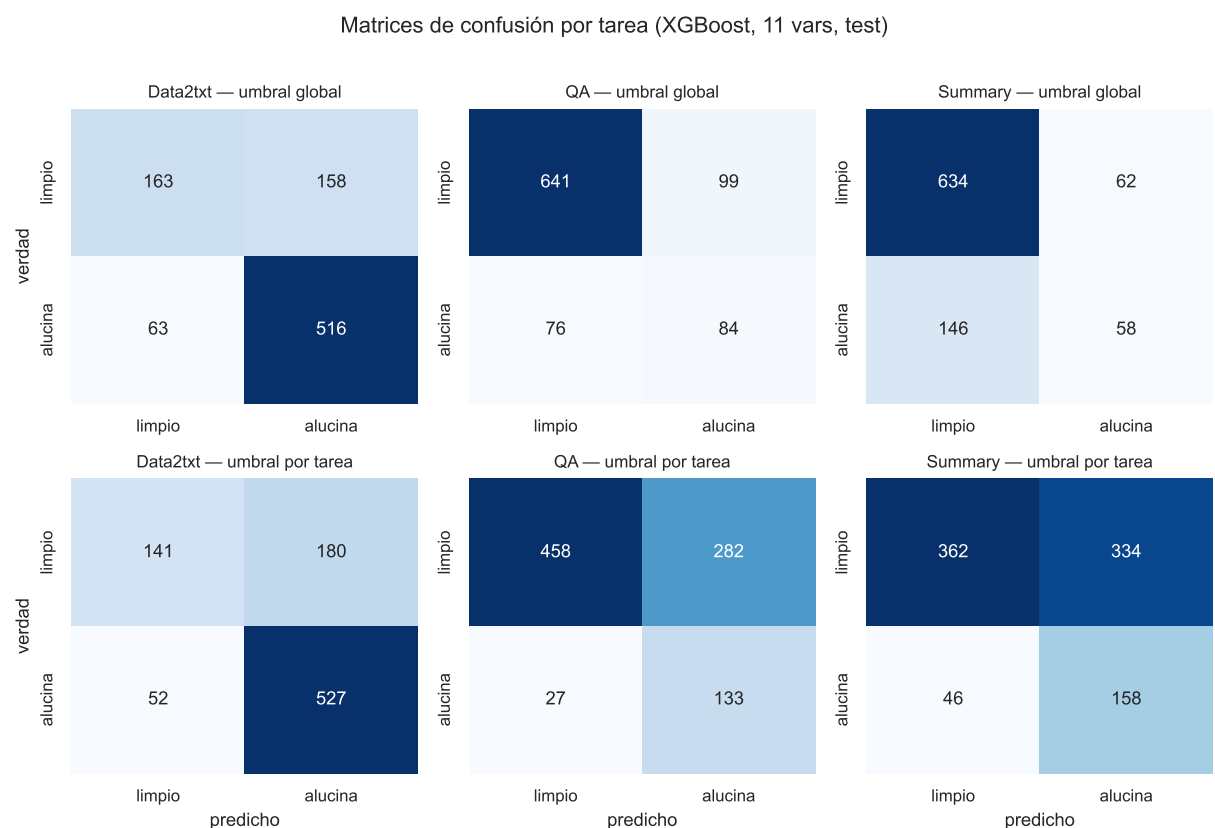
Figura 1.16: Matrices de confusión por tarea (XGBoost, test). Fila superior: umbral global; fila inferior: umbral por tarea. La detección de alucinaciones (VP) crece en QA y Summary.
