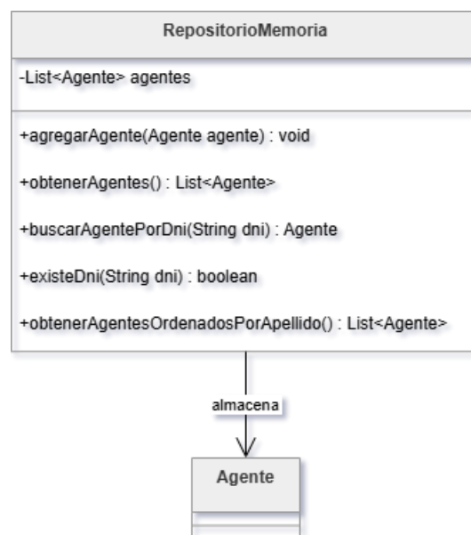
Imagen 40 – Diagrama de Clase RepositorioMemoria
