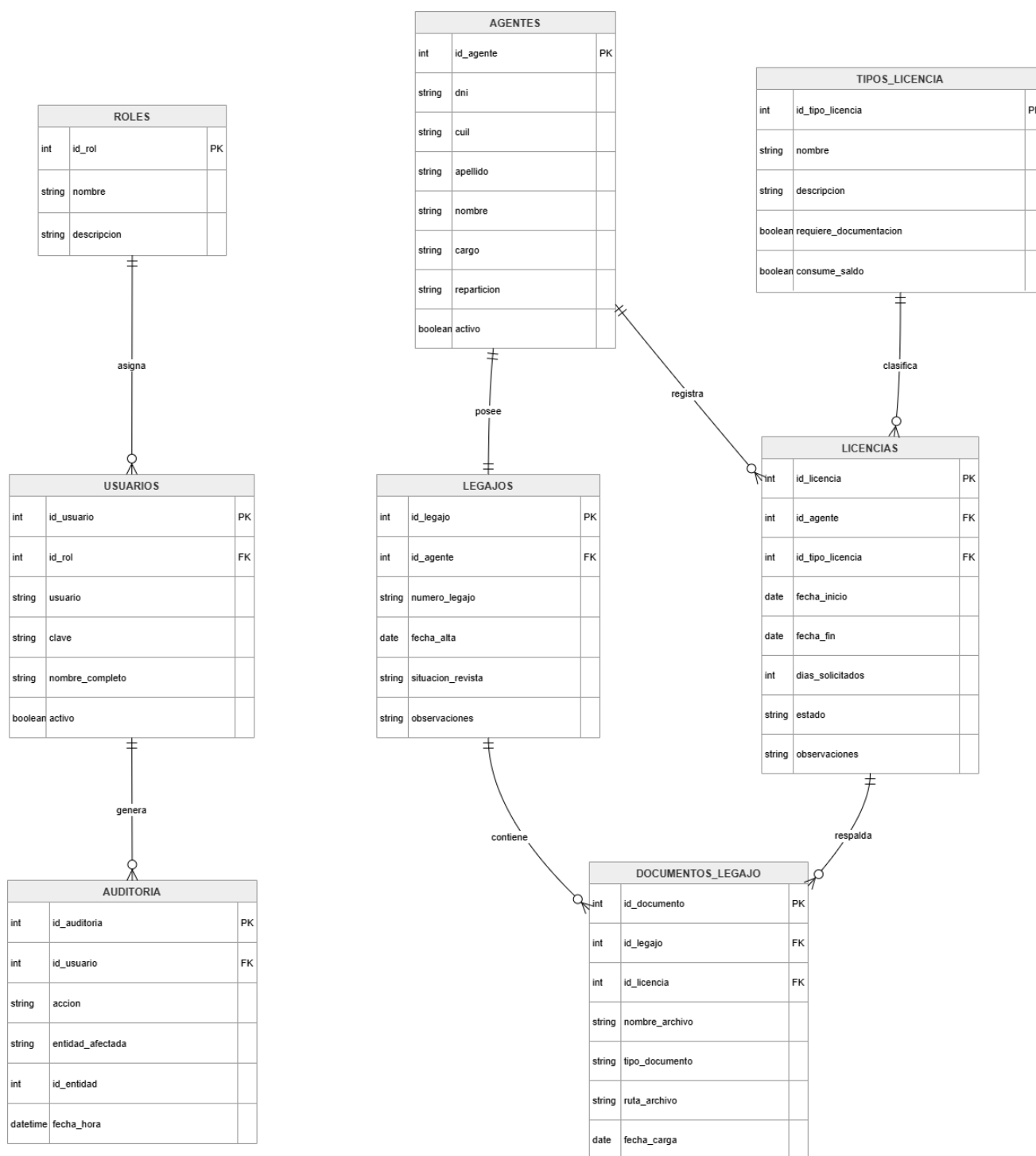
Imagen 19 – Diagrama de Entidad-Relación
