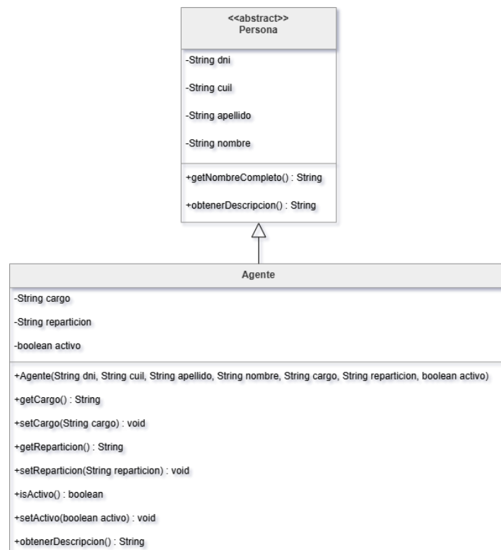
Imagen 38 – Diagrama de Clase Agente
