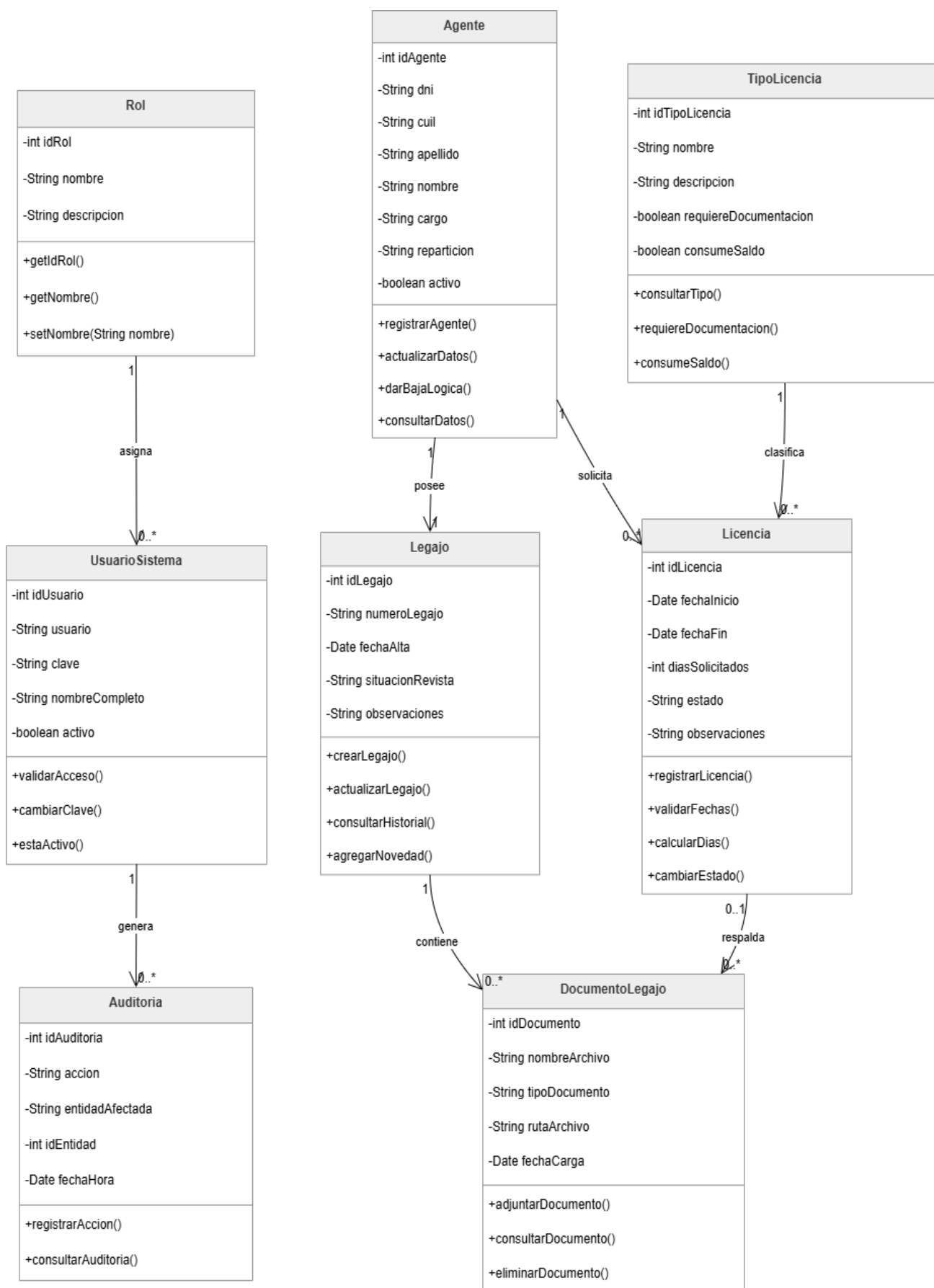
Imagen 10 – Diagrama de clases
