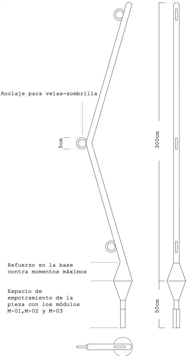
Planta y alzados 1:20
