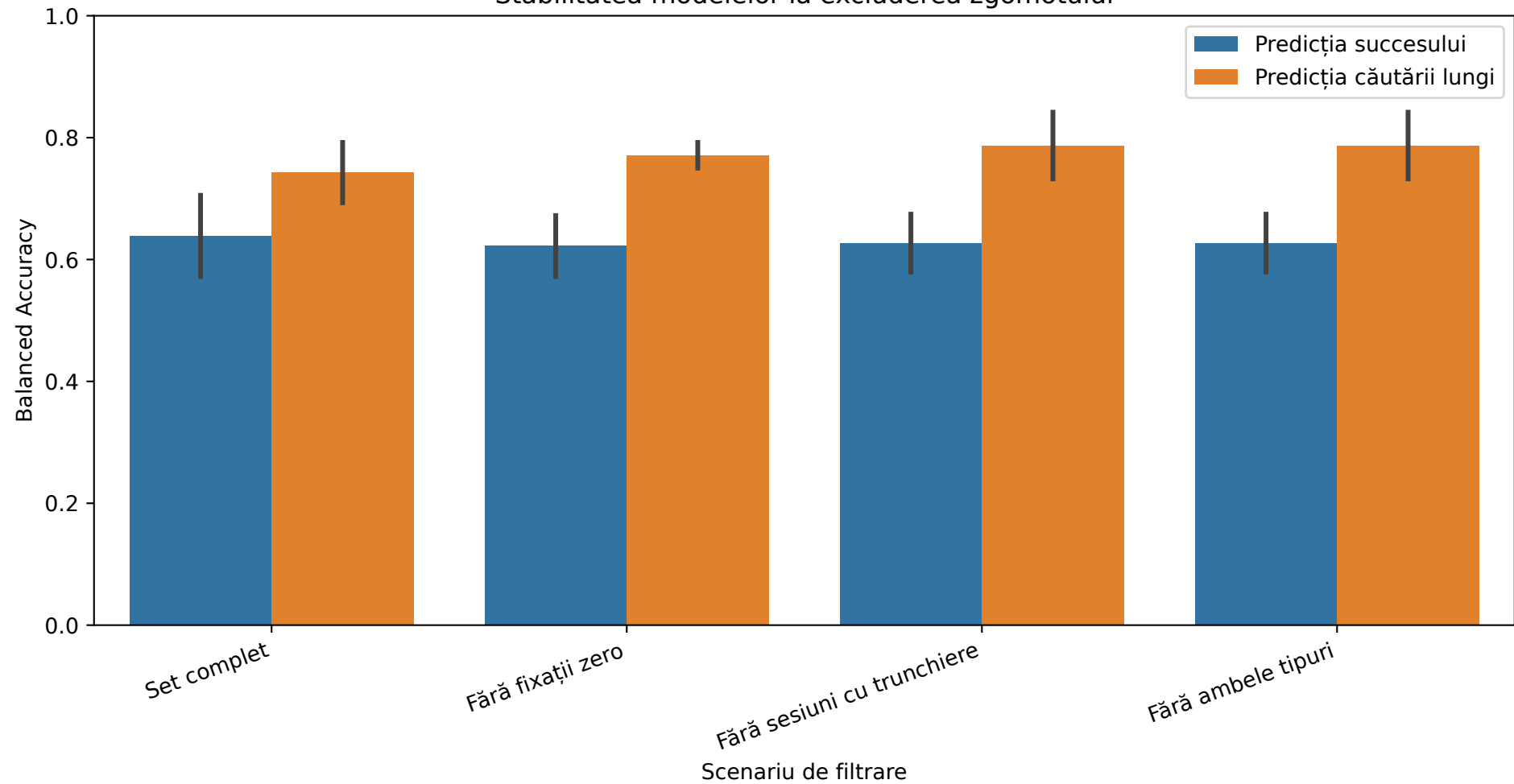
Stabilitatea modelelor la excluderea zgomotului
