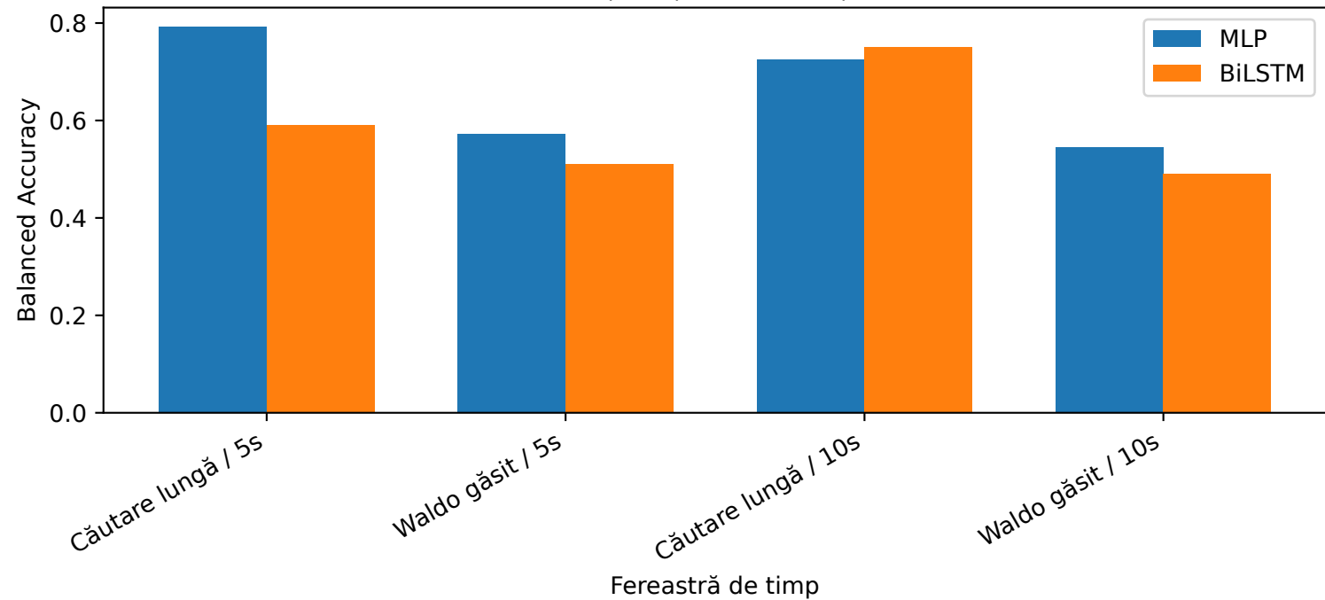
Performanța rețelelor MLP și BiLSTM
