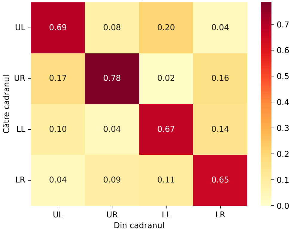
Matricea tranzițiilor: nivelul 2
