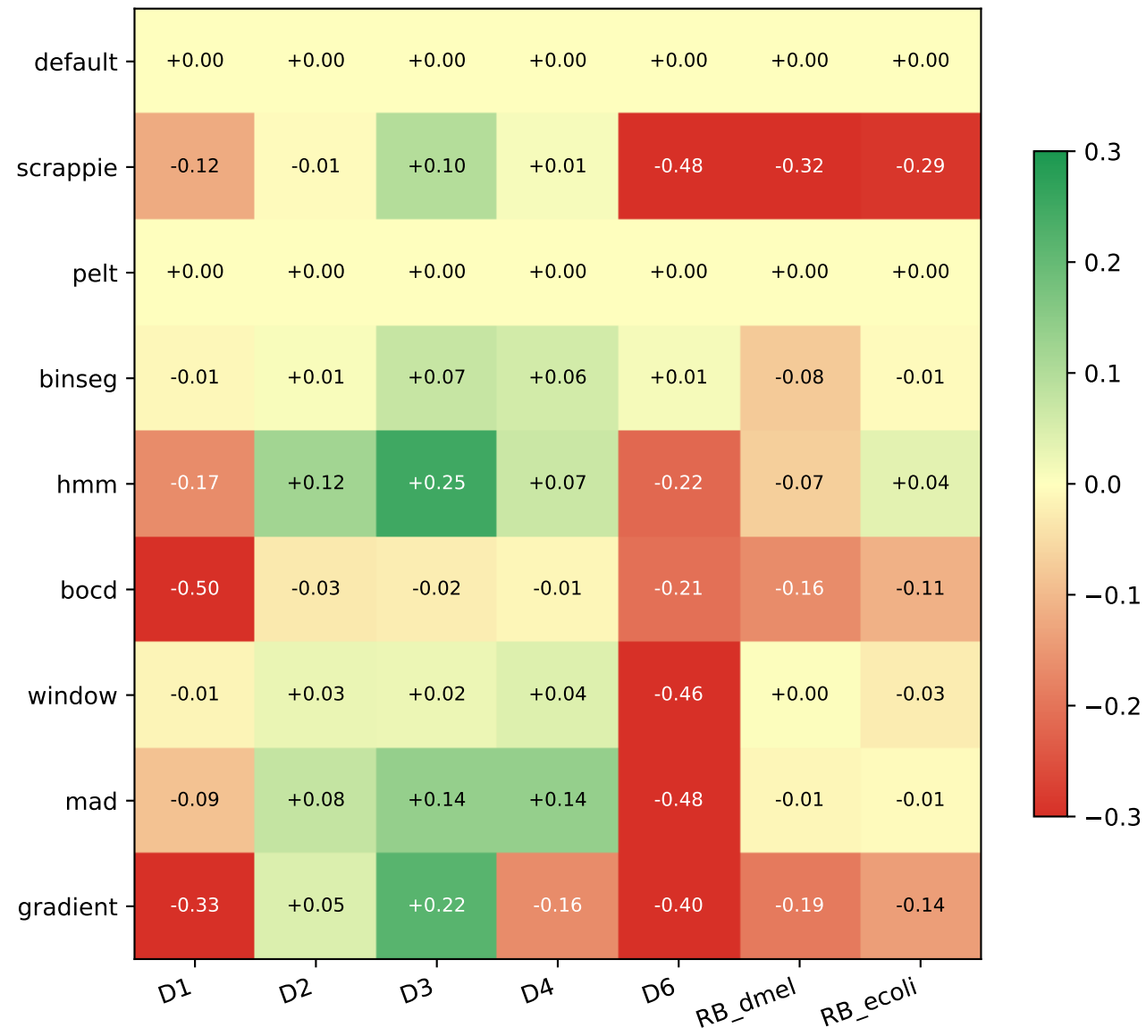
F1 delta vs default
