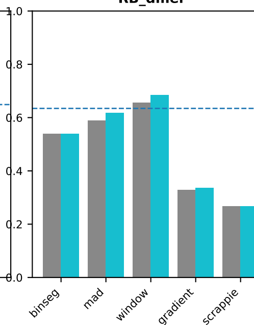
RB_dmel
