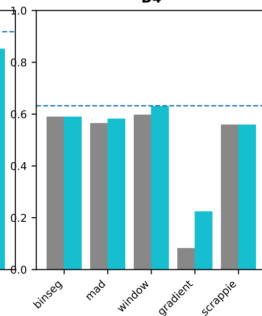
RB_hsap_sub
