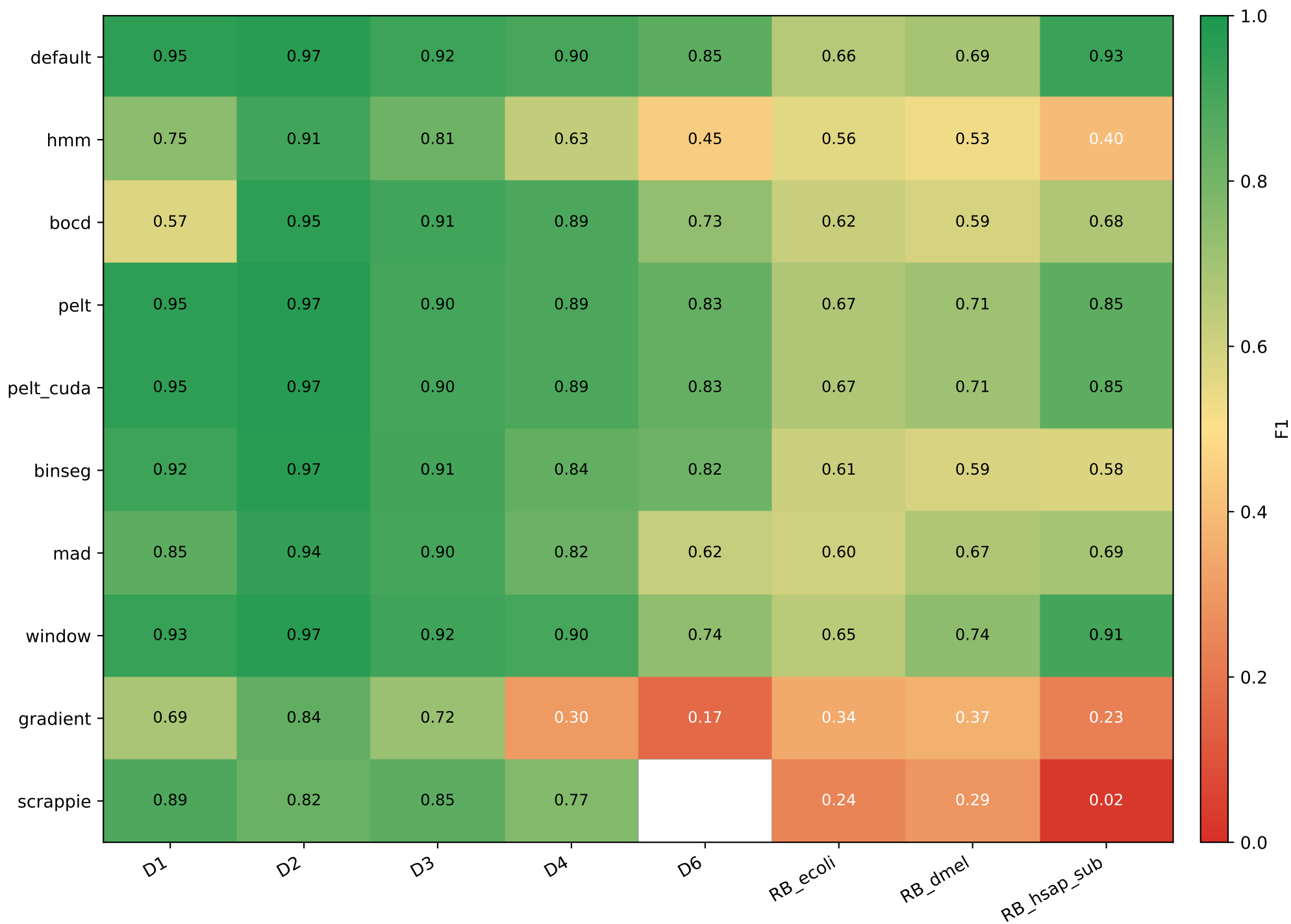
F1 d \leq 100\text{kb} (lenient) — best mode per segmenter
