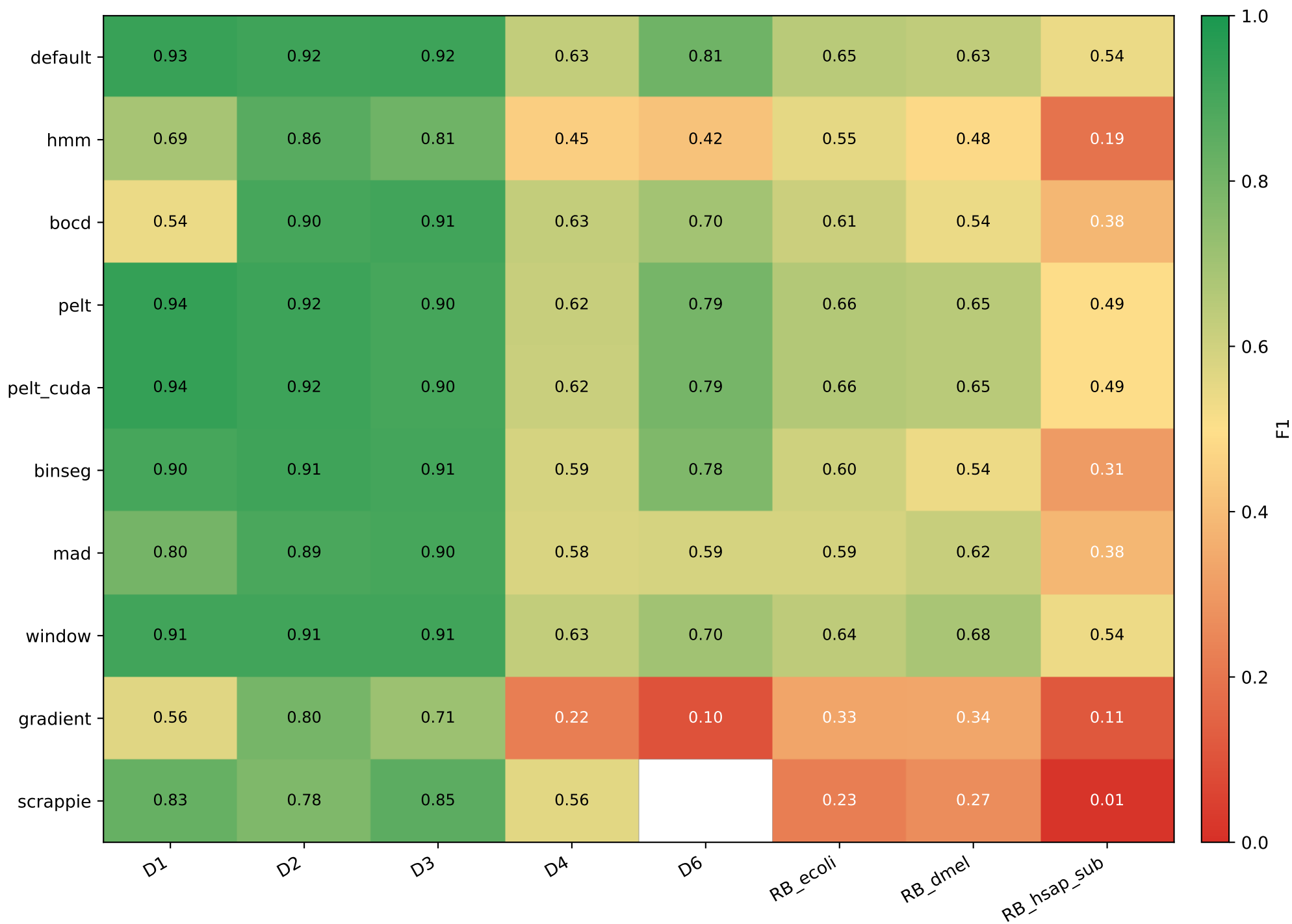
F1 d \leq 10\text{kb} — best of (auto/static) per segmenter
