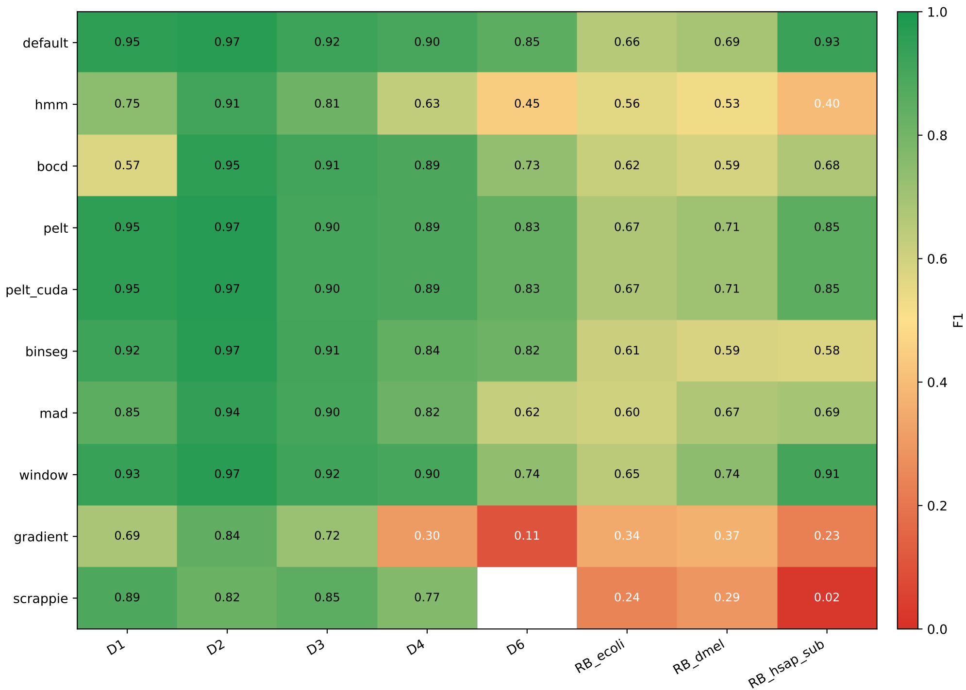
F1 d≤100kb (lenient) — best mode per segmenter
