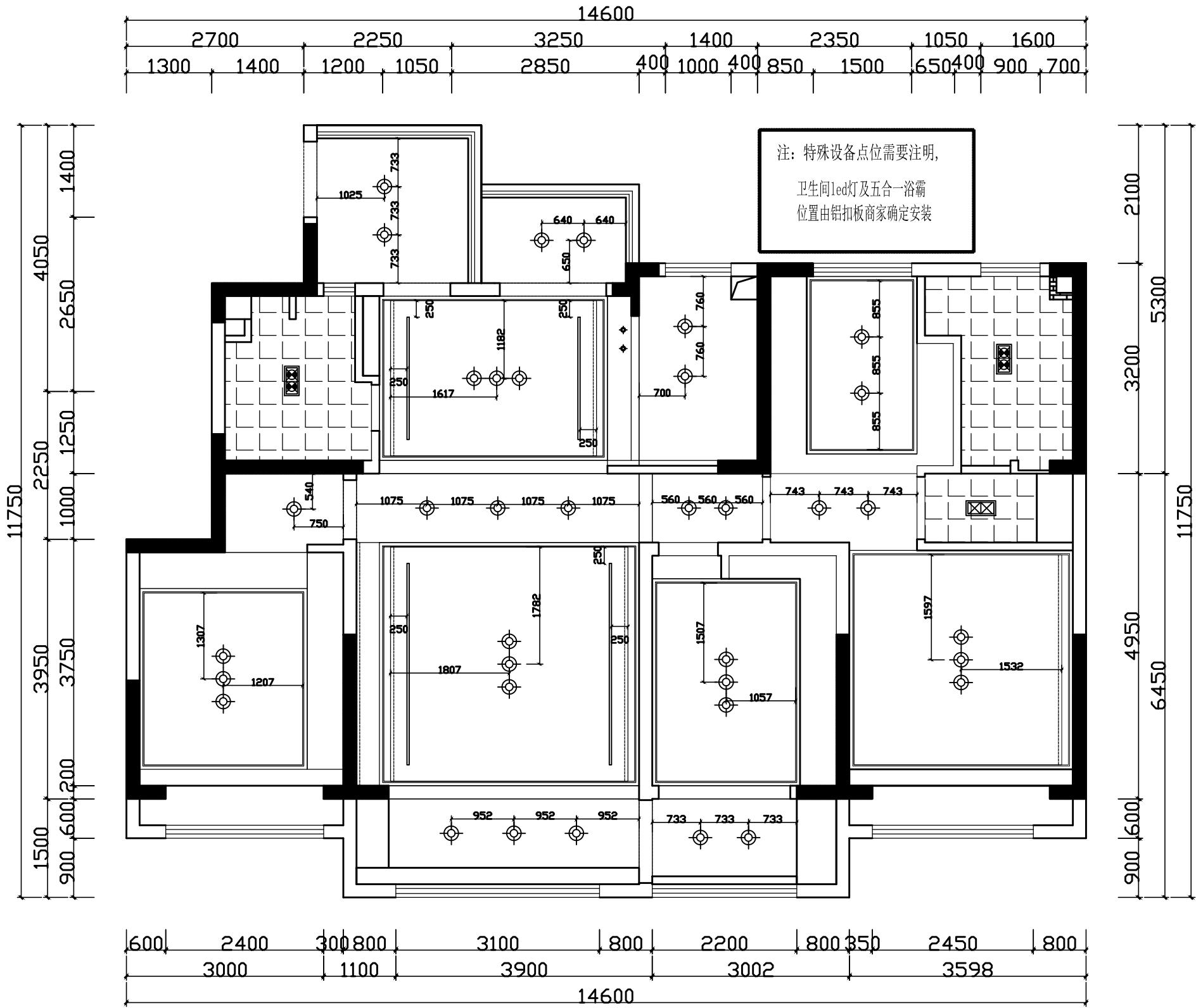
顶面灯具图 原始户型图 SCALE:1/30
