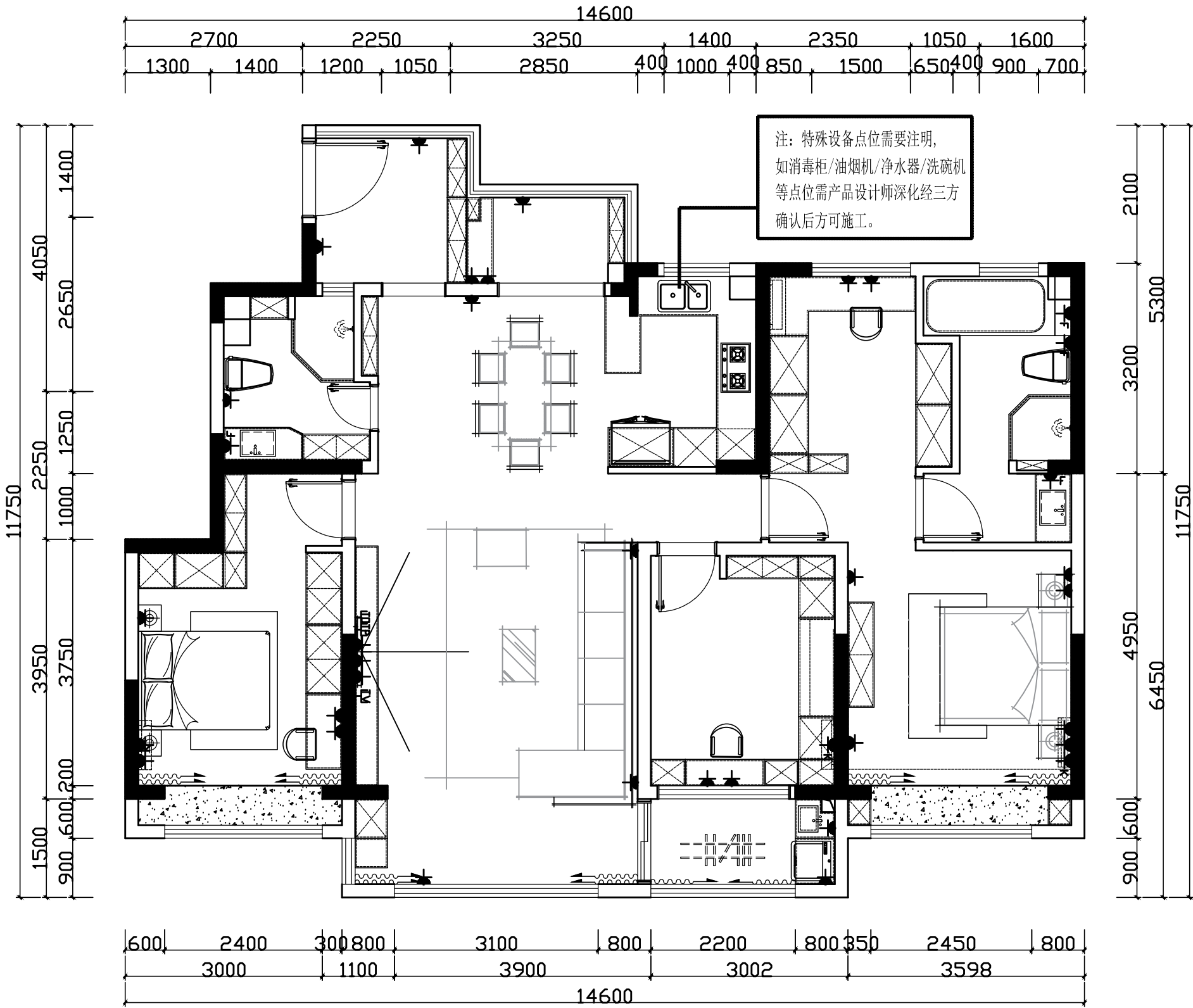
强弱电布置图 平面方案图 SCALE:1/30
