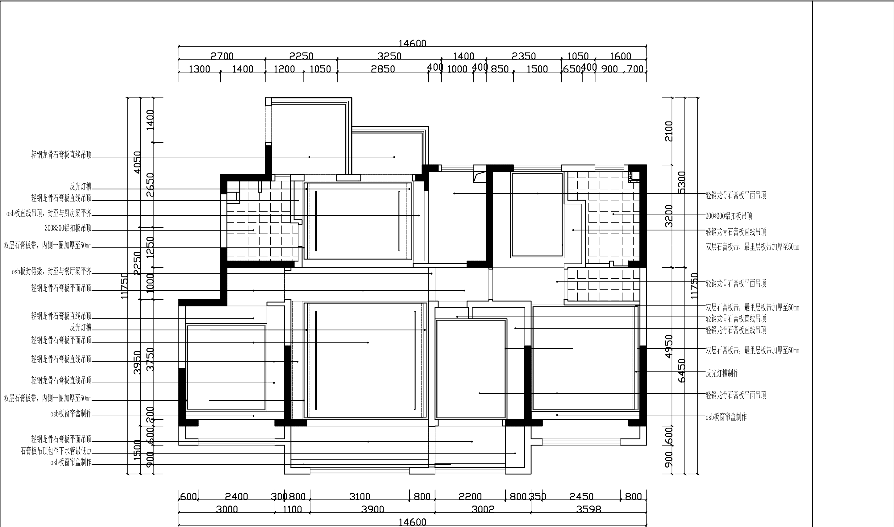
0 顶面吊顶图 08 原始户型图 SCALE: 1/30
