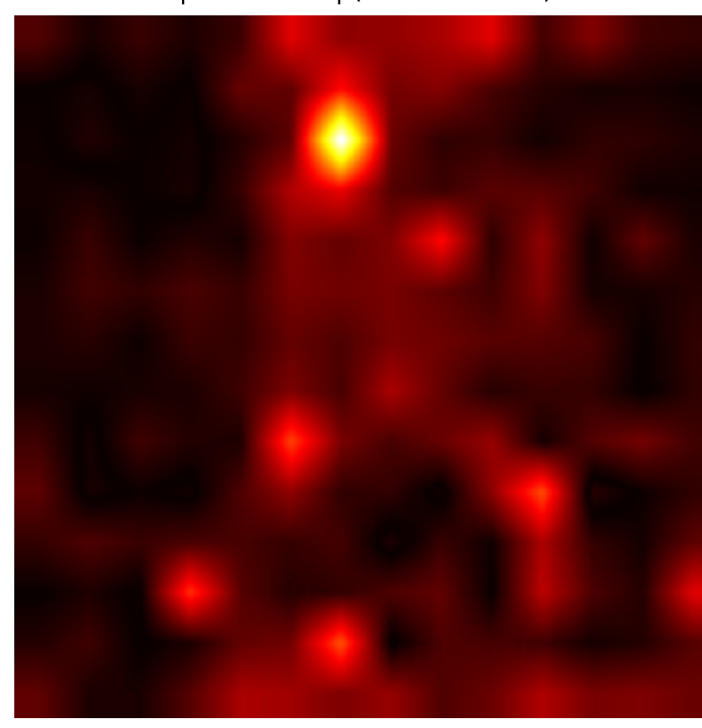
|d-mask224| (max=1.1e-05)
