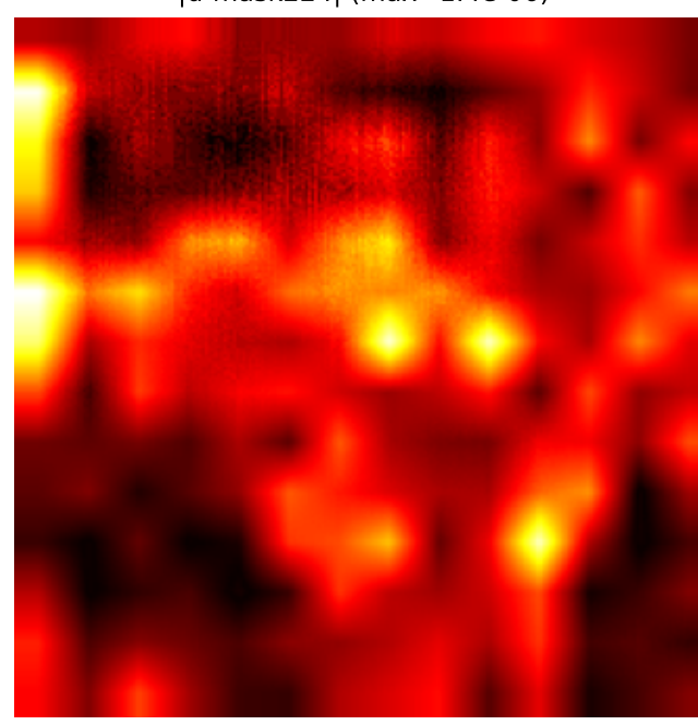
|d-mask224| (max=1.4e-06)
