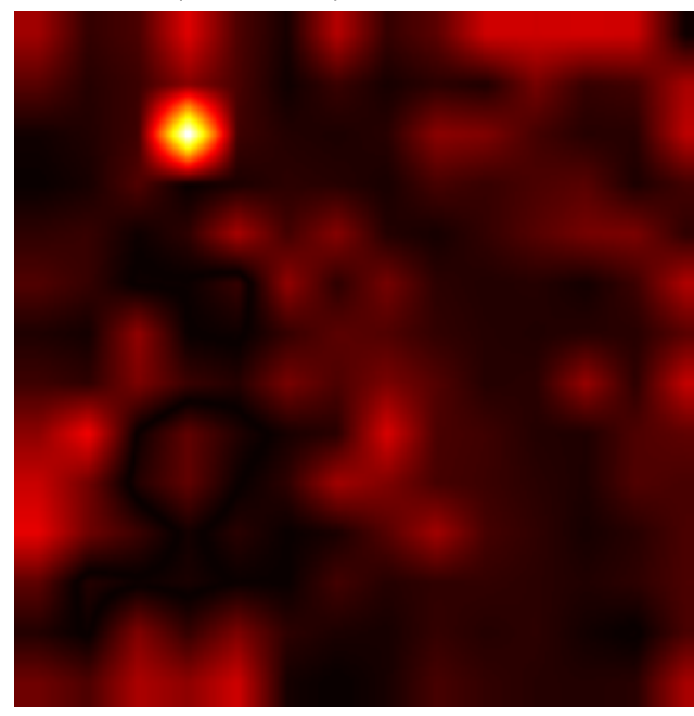
|d-mask224| (max=1.3e-03)
