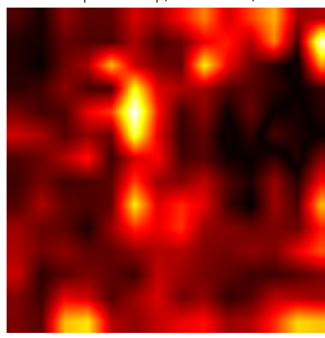
|d-mask224| (max=3.1e-03)
