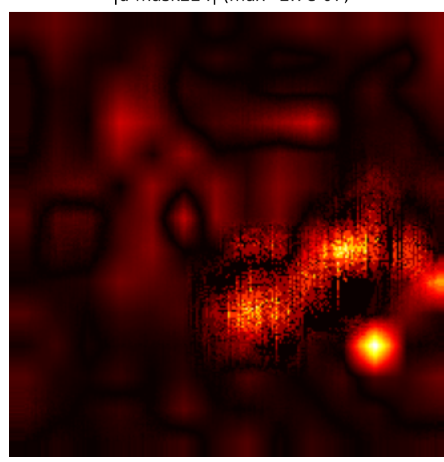
|d-mask224| (max=2.7e-07)
