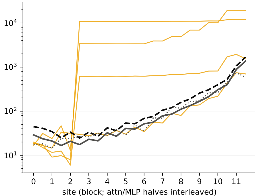
M4 DINOv3-B (+reg, frozen bb) · ImageNet
