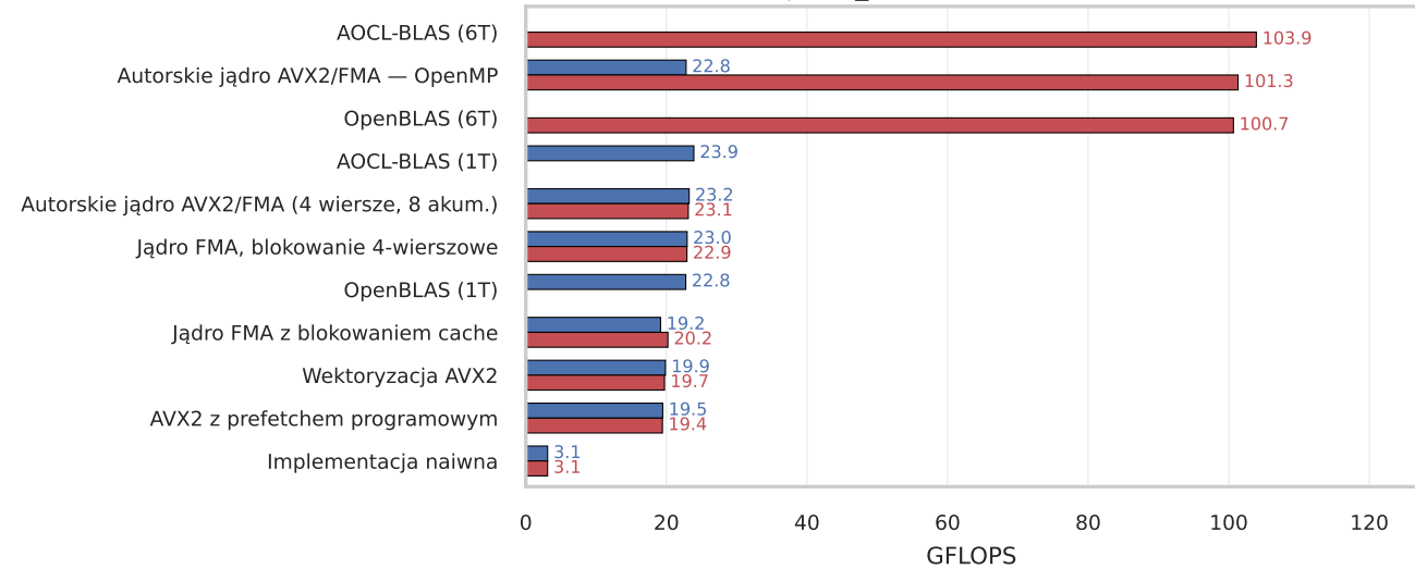
gemv_medium (1024x1024)
