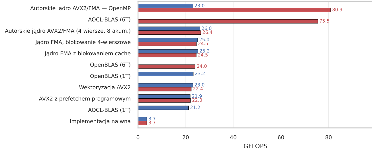
gemv_small (256x256)
