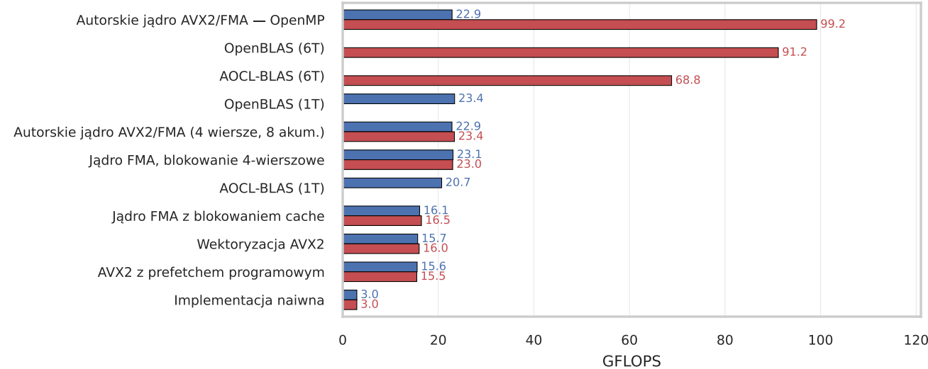
gemv_wide (256x8192)
