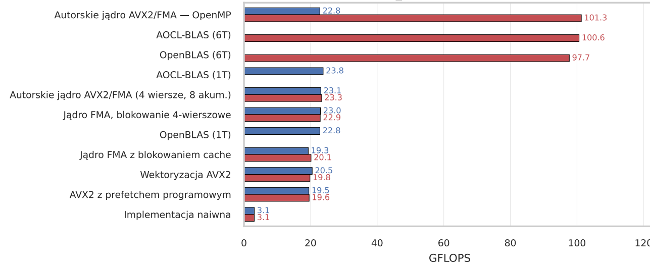
gemv_medium (1024x1024)
