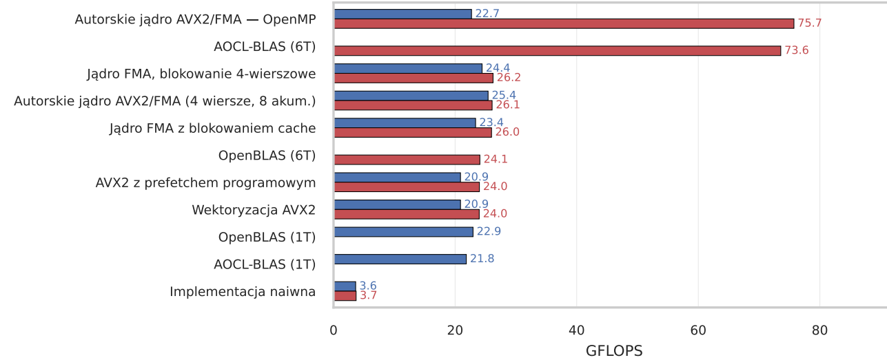
gemv_small (256x256)
