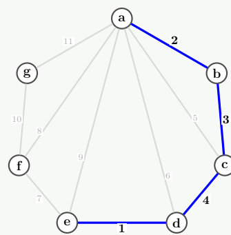
Step 4: Add cd(4)
