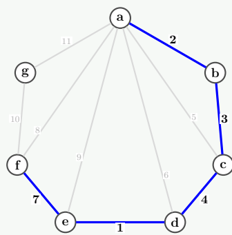
Step 5: Skip ac , ad . Add ef(7)
