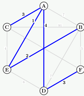
Step 5: Add DA(4)
