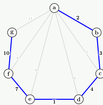
Step 6: Skip af , ae . Add fg(10)
