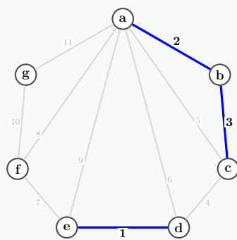
Step 3: Add bc(3)
