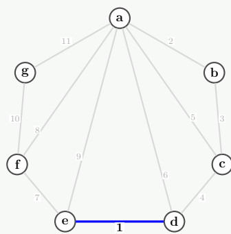
Step 1: Add de(1)
