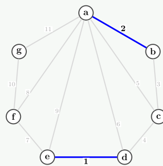
Step 2: Add ab(2)
