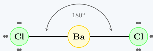
Linear ( sp )
