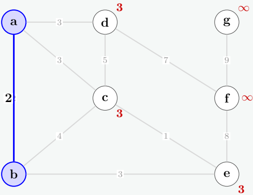
Step 1: Add b
