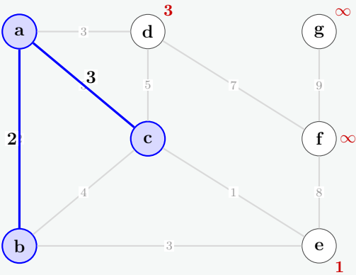
Step 2: Add c
