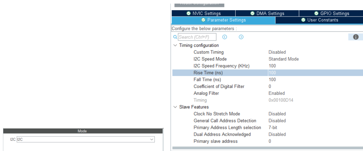
Figura 3: Configuración de I2C1 en STM32CubeMX: modo de funcionamiento y parámetros de transferencia.
