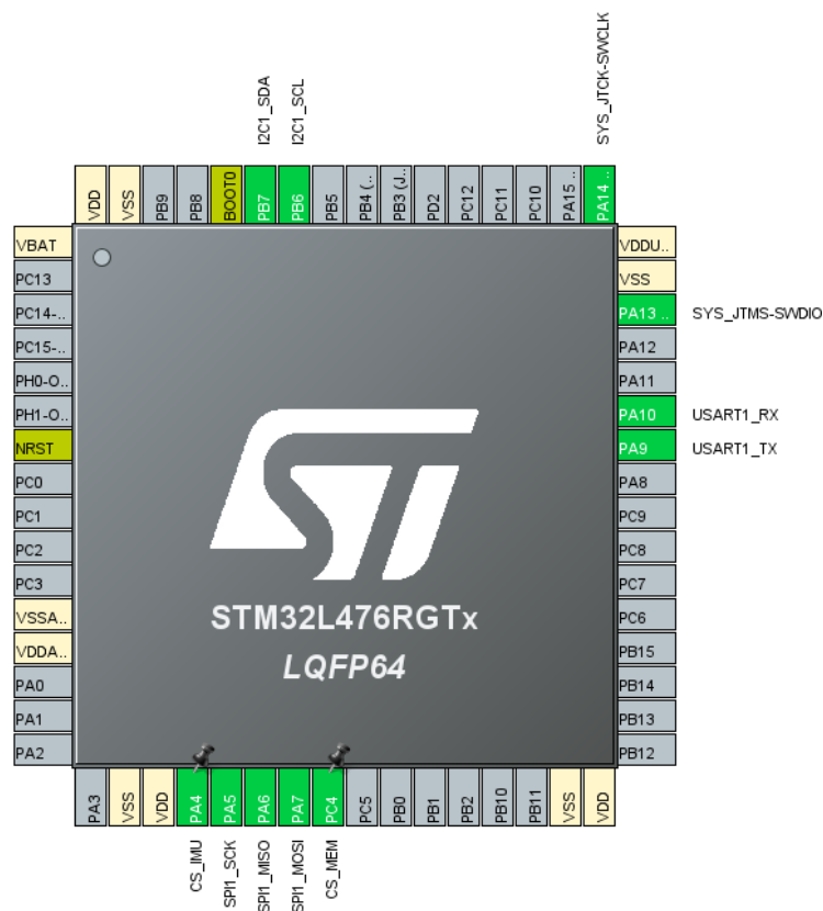
Figura 1: Asignación de pines del STM32L476RGT6 realizada en STM32CubeMX.
