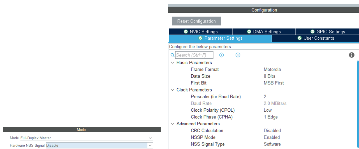
Figura 2: Configuración de SPI1 en STM32CubeMX: modo de funcionamiento y parámetros de transferencia.
