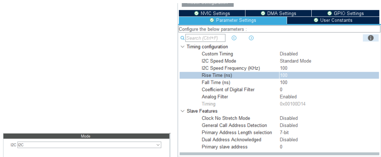
Figura 3: Configuración de I2C1 en STM32CubeMX: modo de funcionamiento y parámetros de transferencia.
