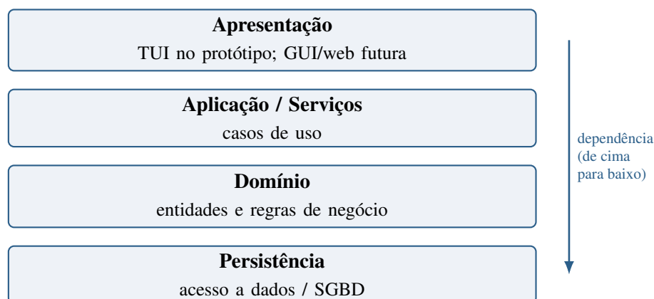
Figura 1: Arquitetura em camadas do ParaFazer
