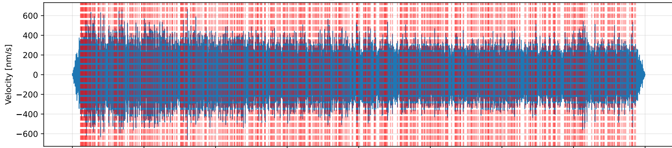
STA_LTA | 0.1-0.3Hz
