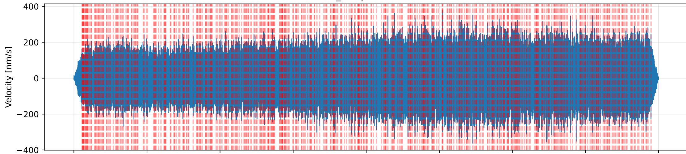
STA_LTA | 0.3-1.0Hz
