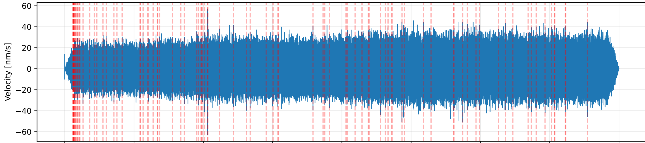
STA_LTA | 1.0-3.0Hz
